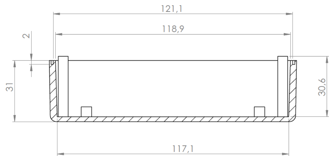
Sección/ Section Z-Z
