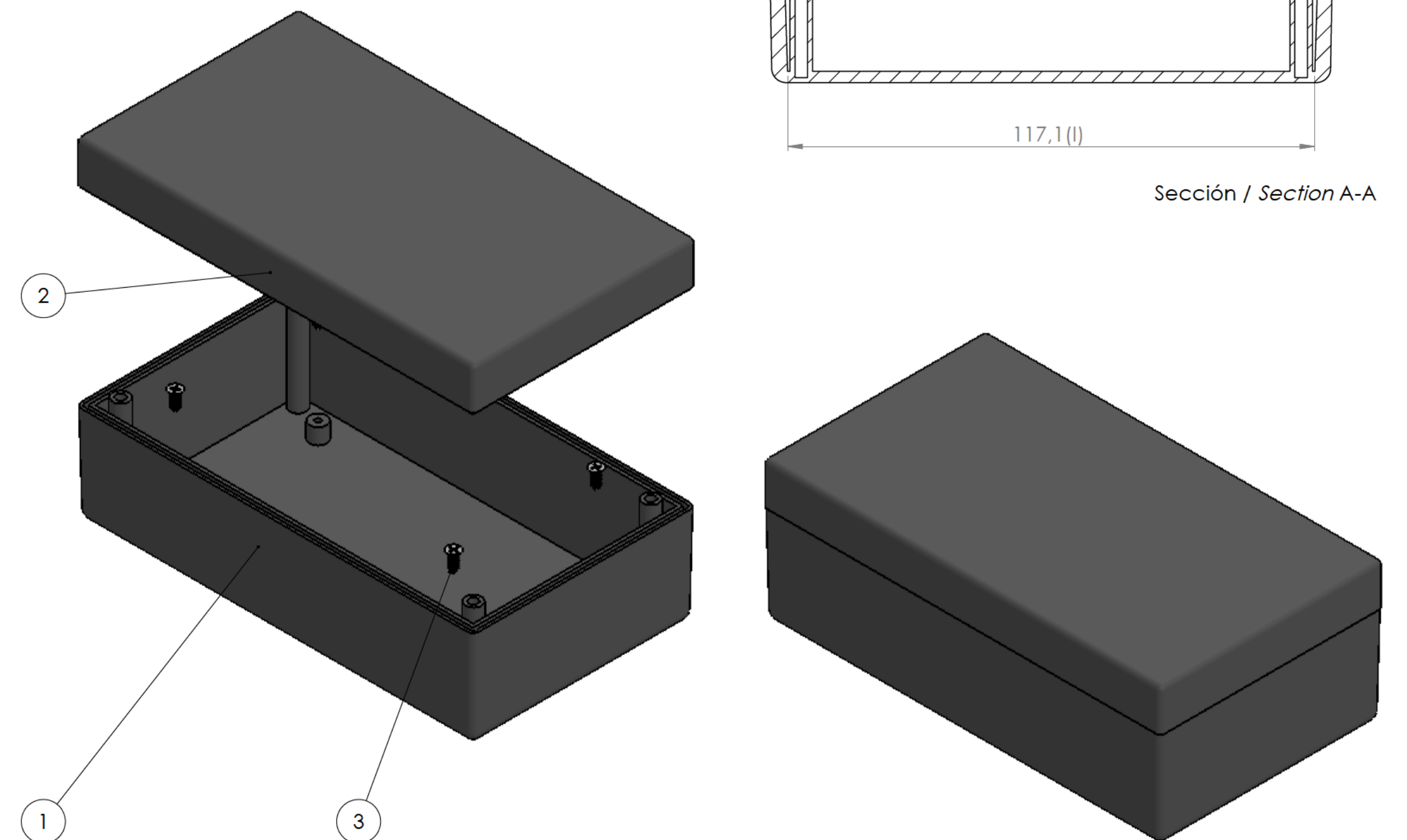
Conjunto Assembly
