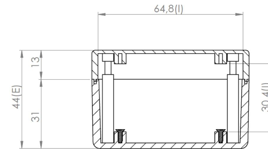
Sección/Section U-U
