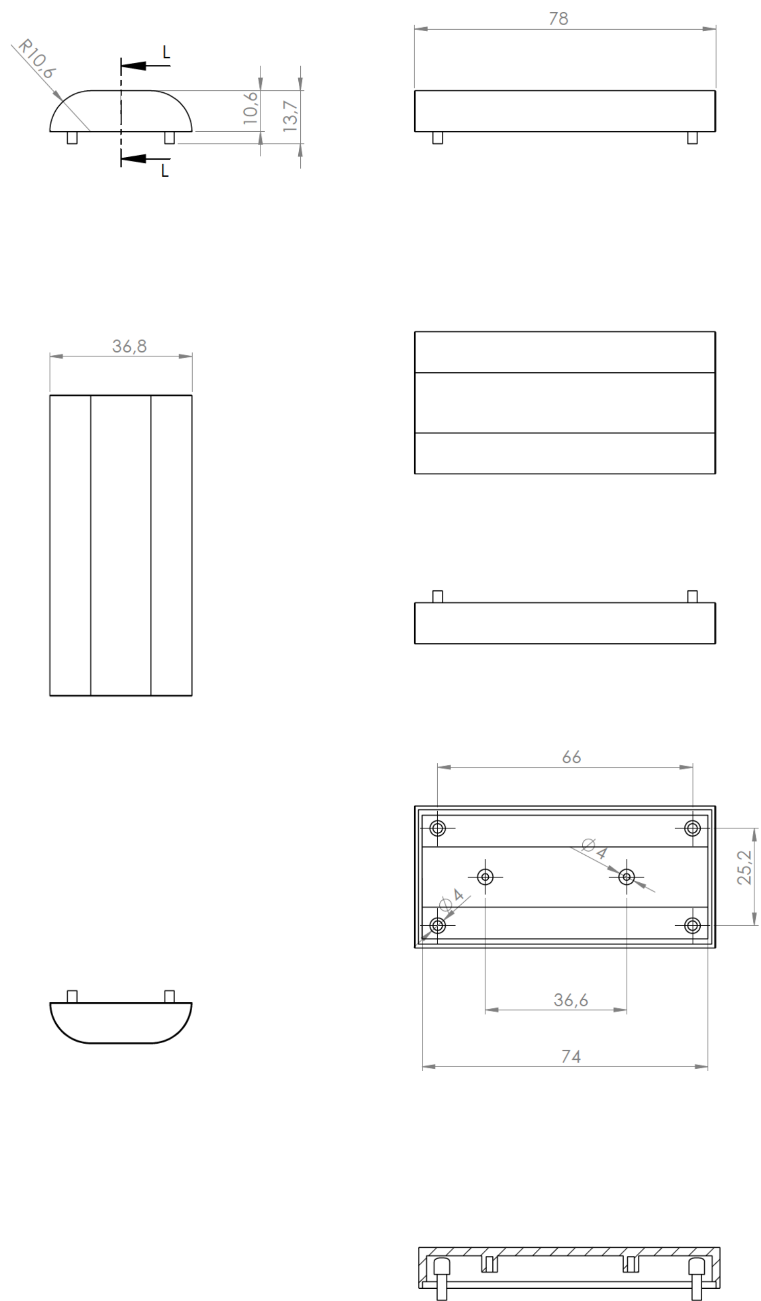
Sección / Section L-L
