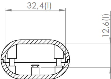
Sección / Section N-N
