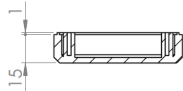
Sección/Section T-T
