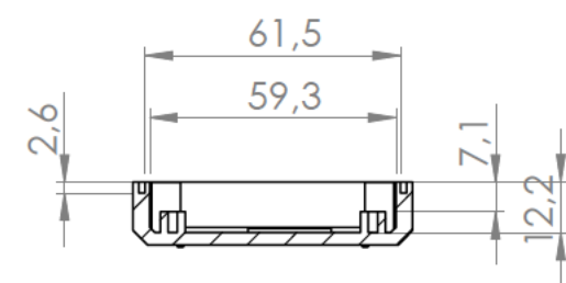
Sección/Section Q-Q
