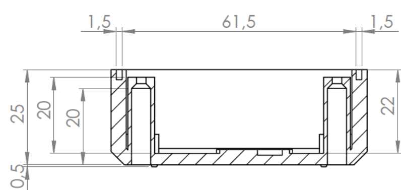
Sección/Section L-L
