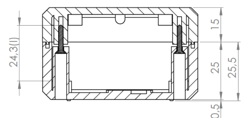
Sección/Section P-P
