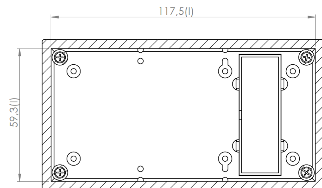
Sección/Section Q-Q
