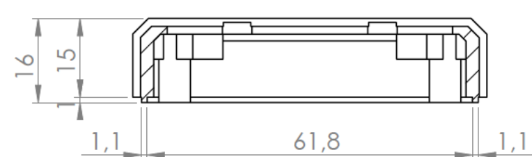
Sección/Section O-O
