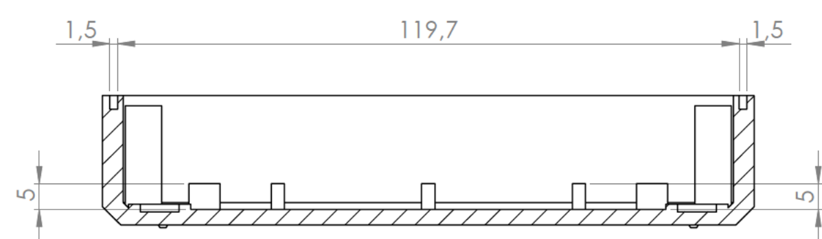
Sección/Section M-M
