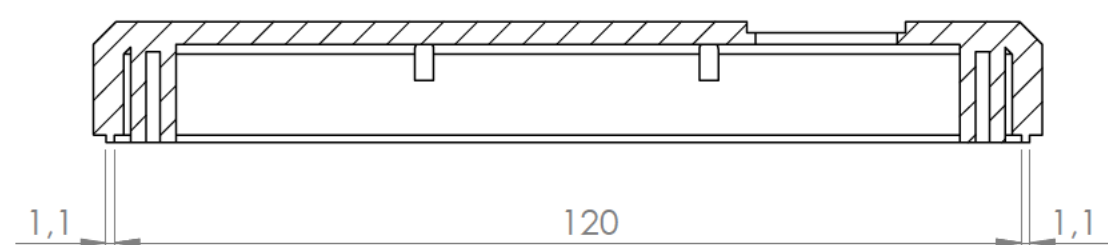
Sección/Section N-N
