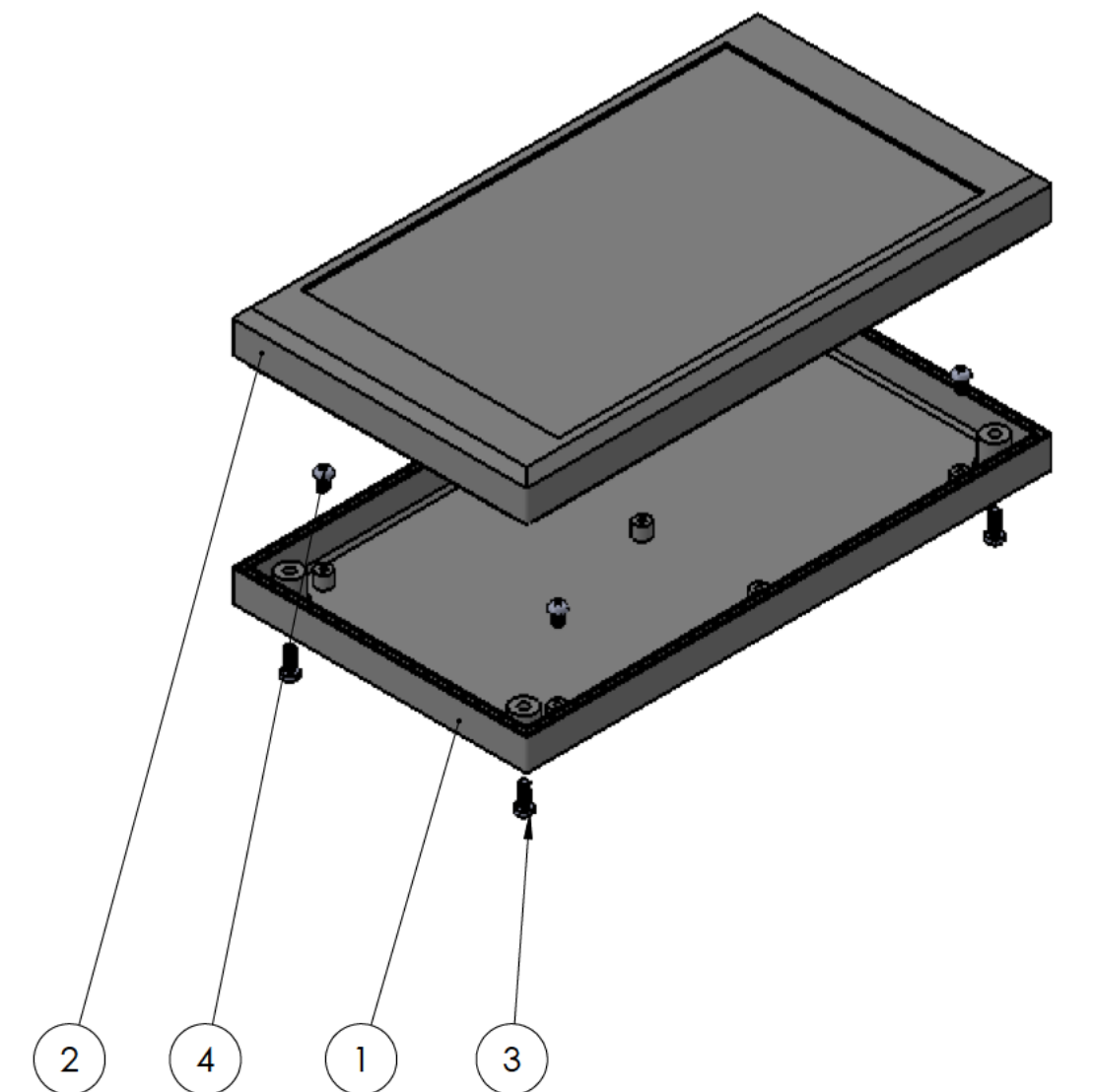
Conjunto Assembly
