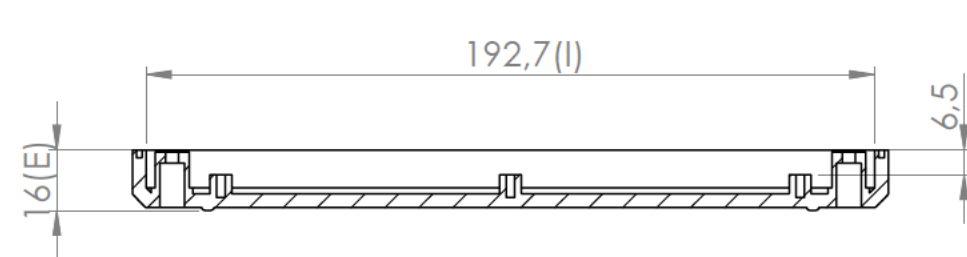
Sección/Section T-T Escala/Scale 1 : 2
