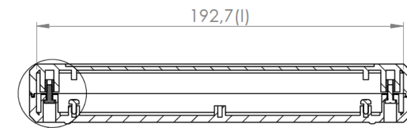
Sección/Section P-P Escala/Scale 1 : 2
