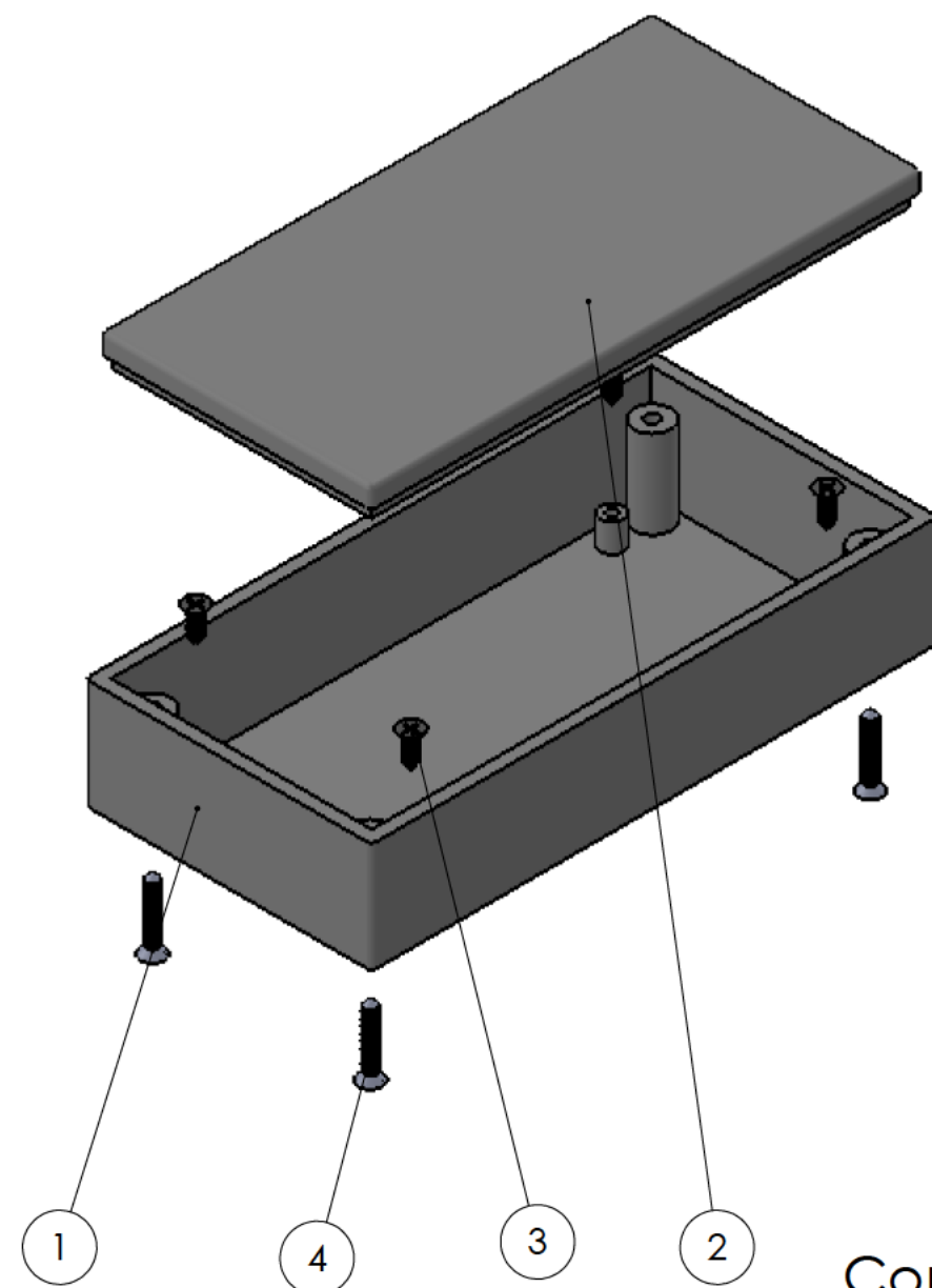
Conjunto Assembly
