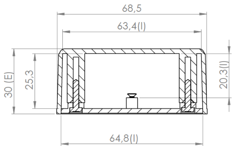
Sección/Section M-M
