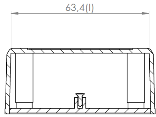
Sección/Section O-O
