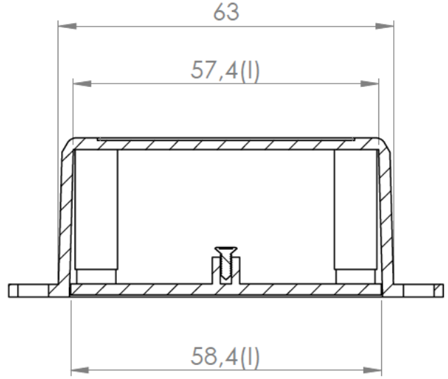
Sección/Section N-N
