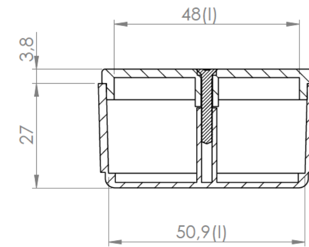
Sección/Section U-U
