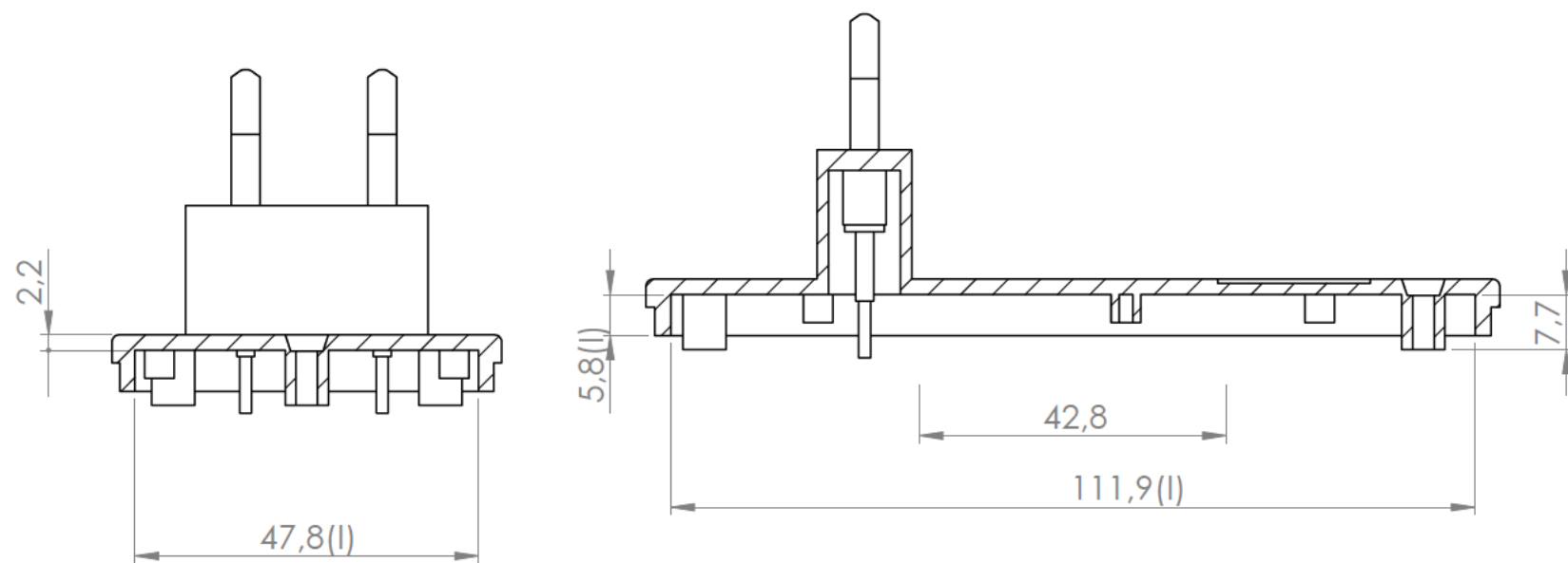
Sección/Section L-L Escala/Scale
