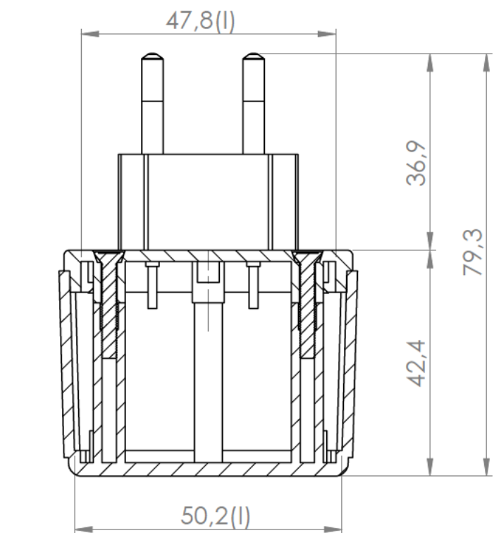
Sección/Section Q-Q
