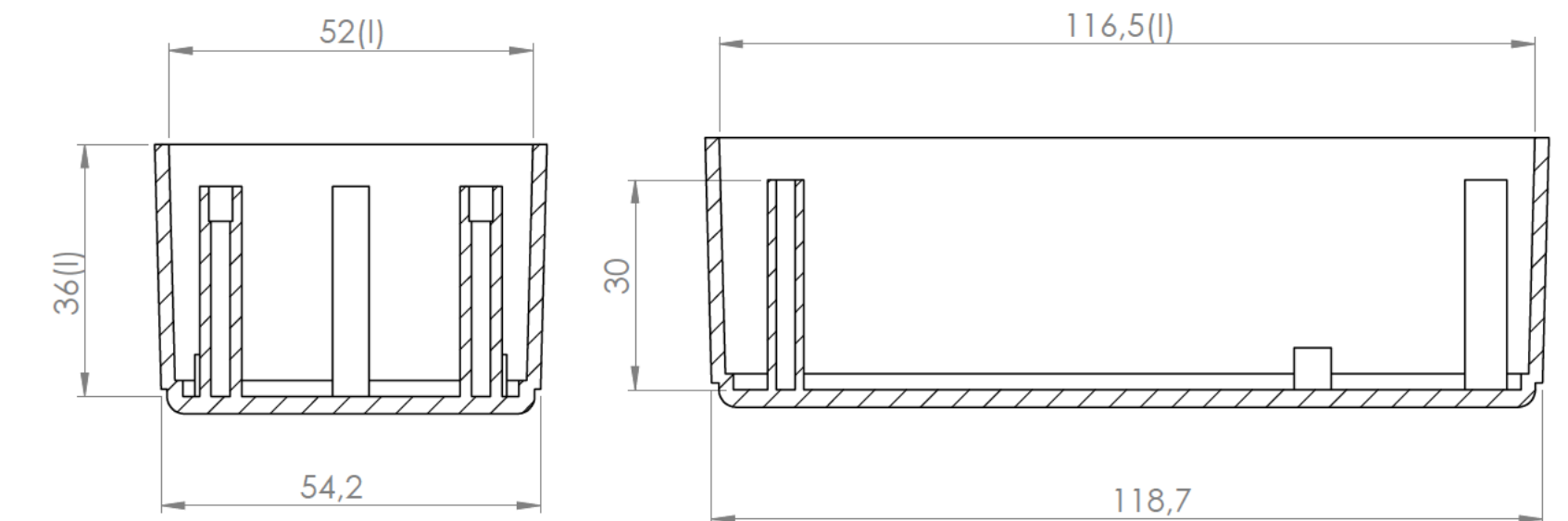
Sección/Section S-S
