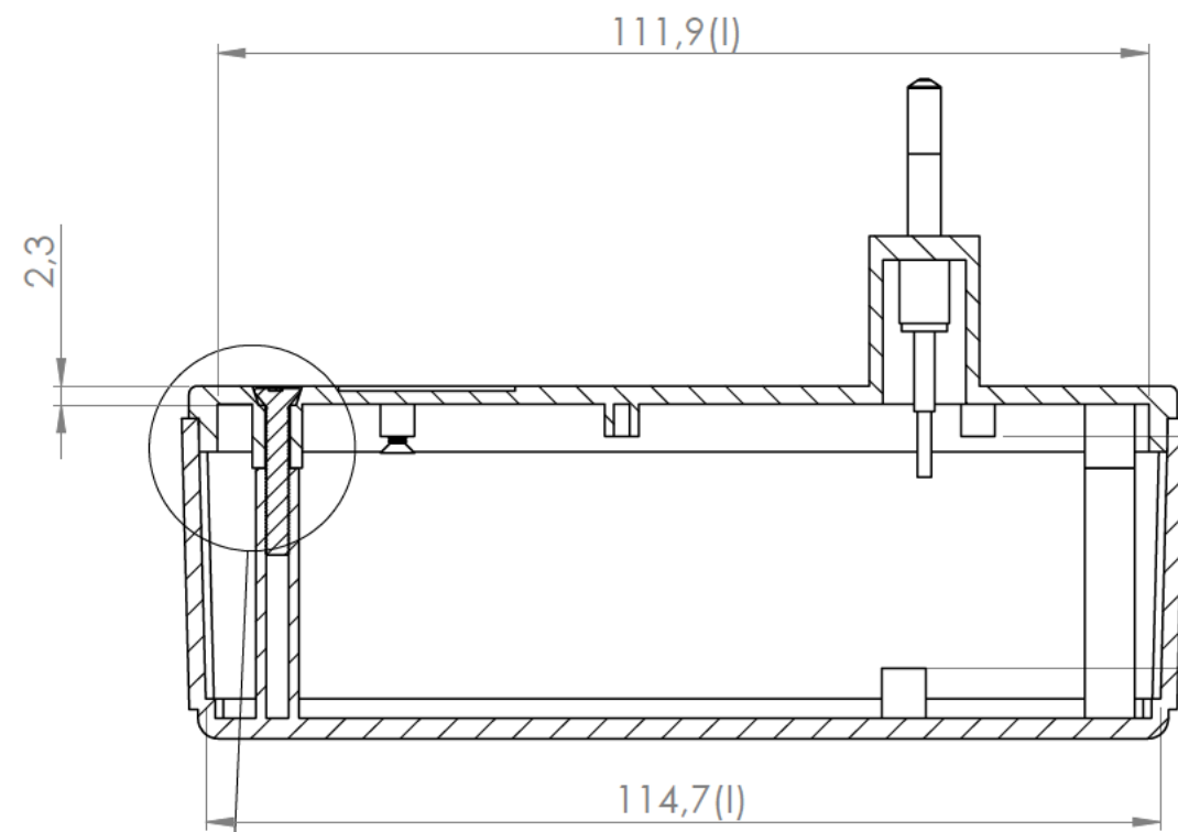
Sección/Section P-P
