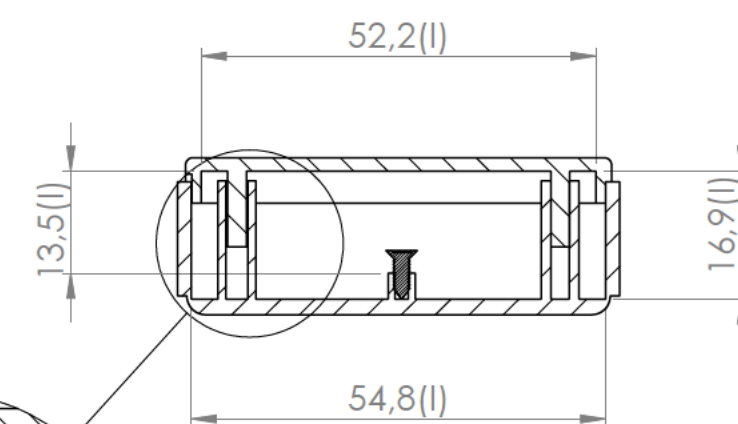
Sección/Section P-P
