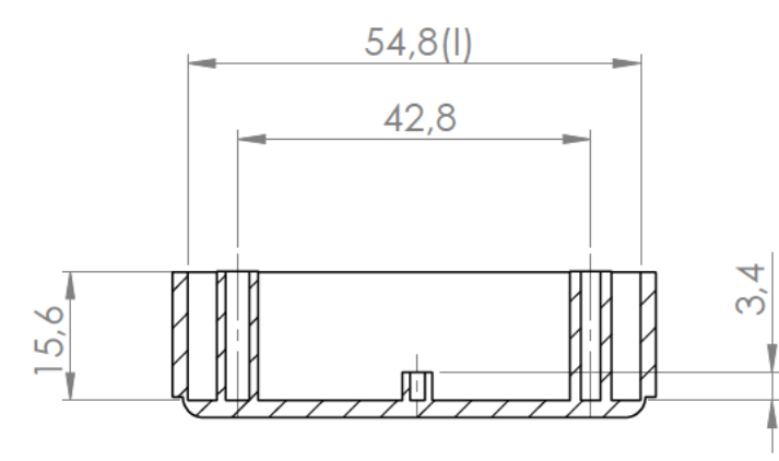
Sección/Section T-T Escala/Scale
