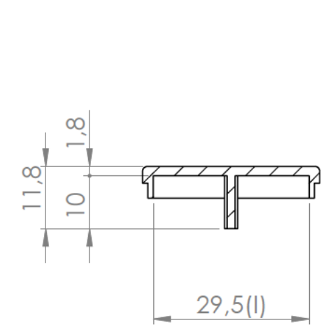
Sección/Section L-L Escala/Scale
