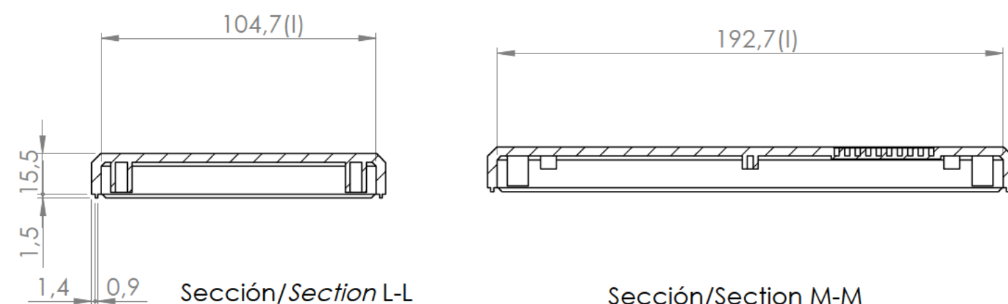
Sección/Section L-L
