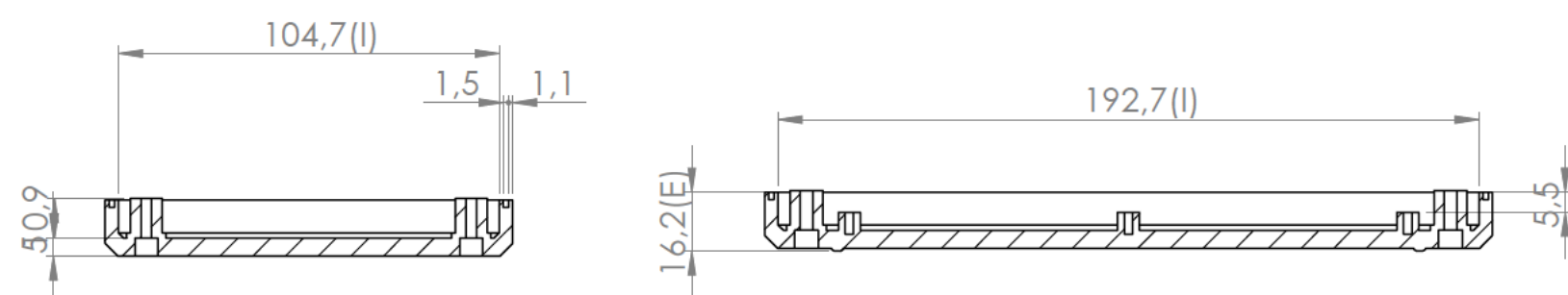
Sección/Section T-T
