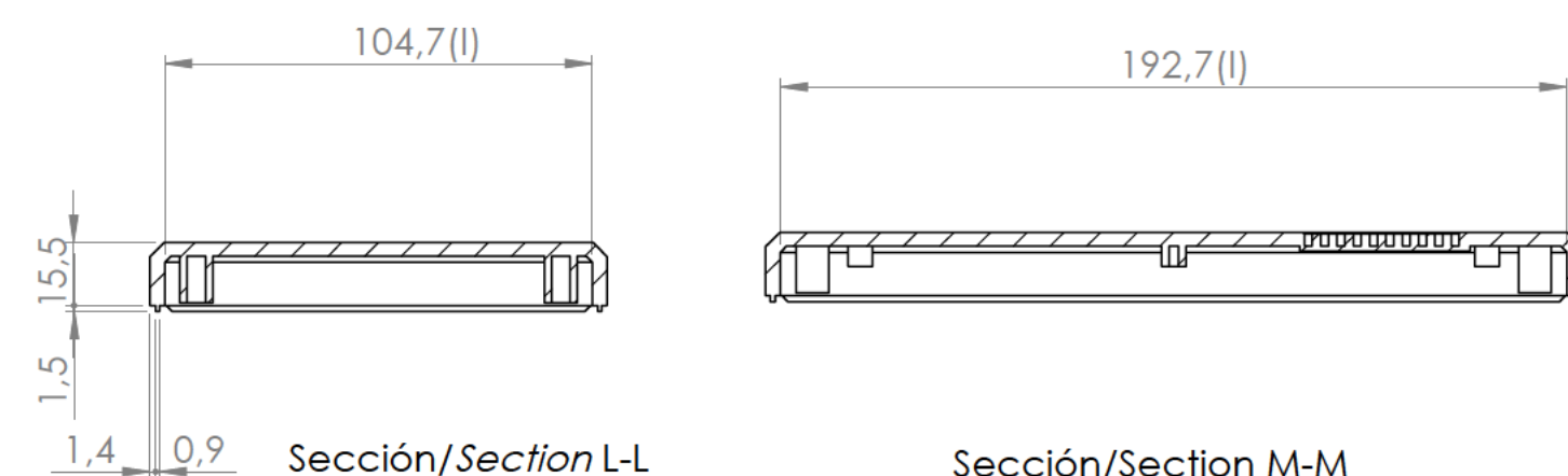
Sección/Section L-L
