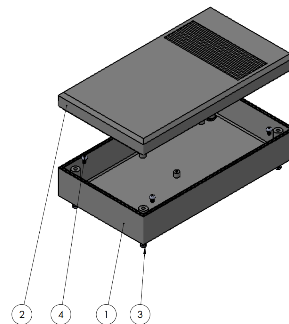
Conjunto Assembly
