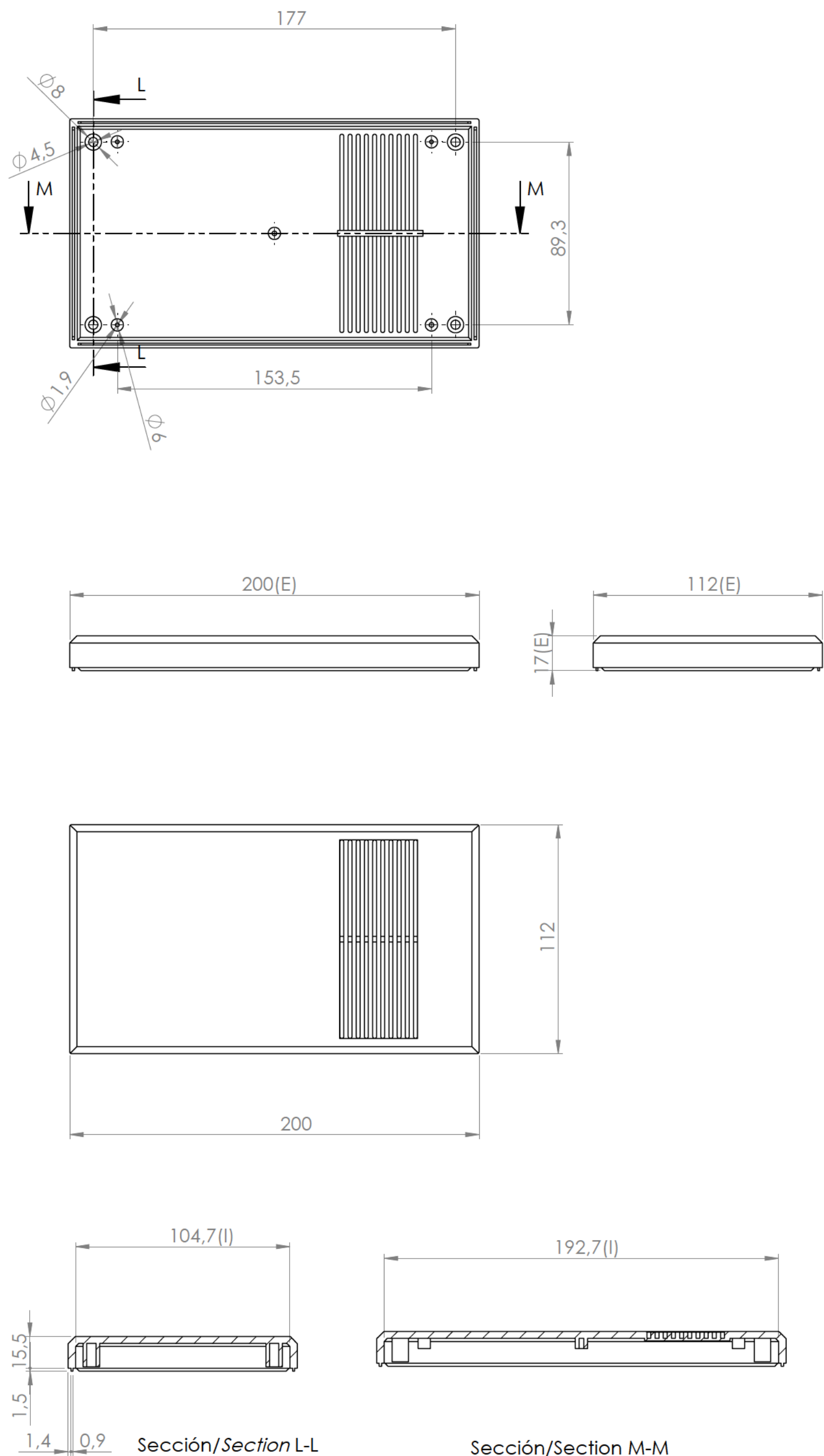
Sección/Section L-L
