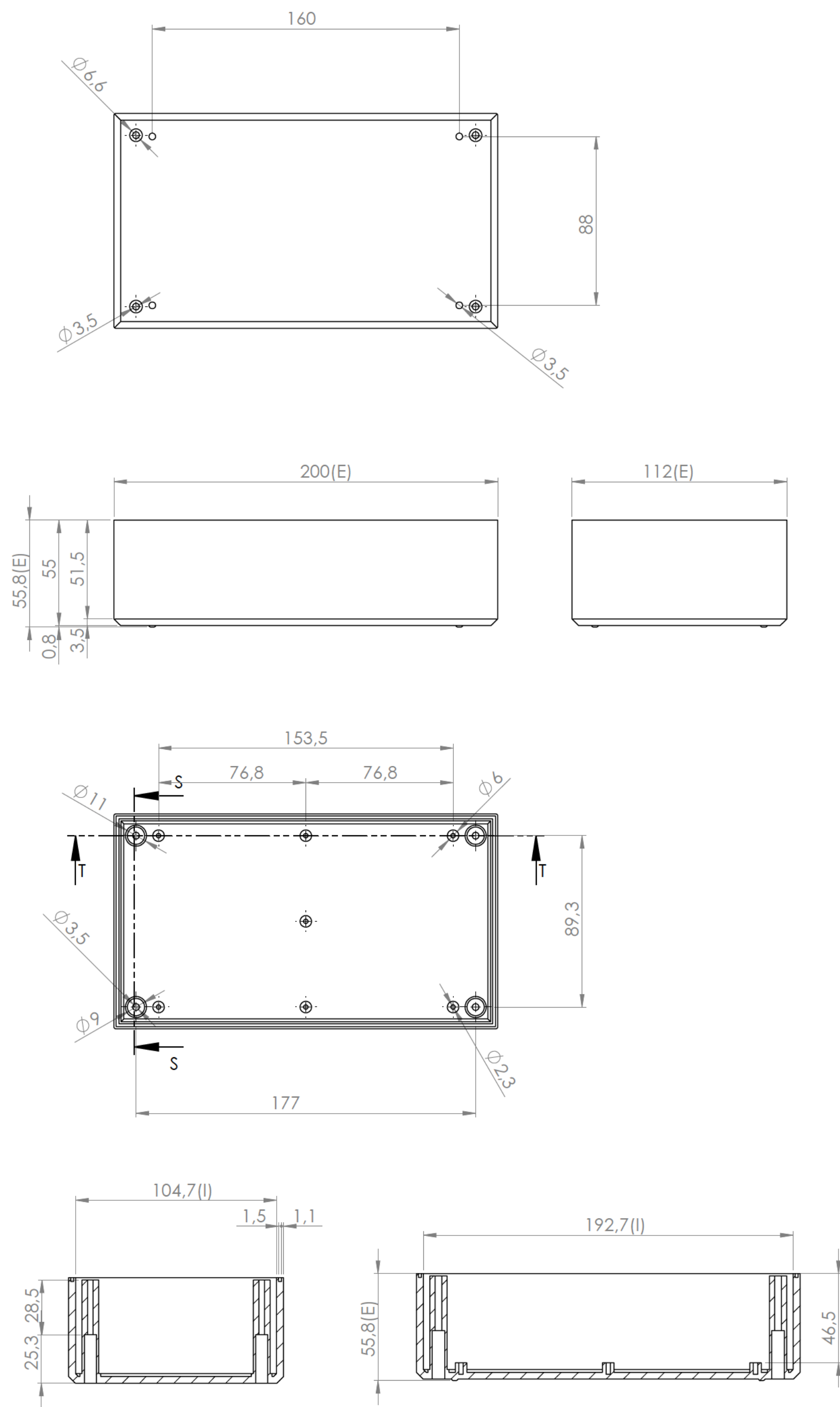
Sección/Section T-T
