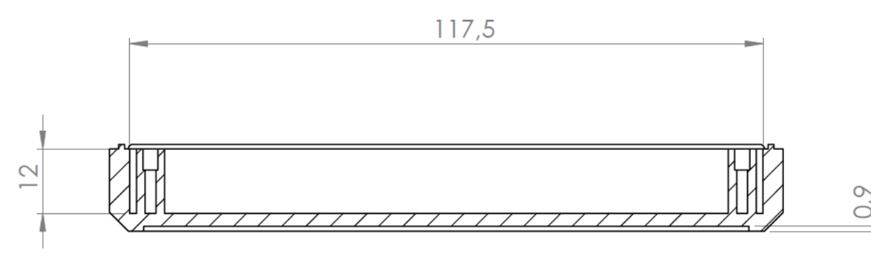
Sección/Section X-X
