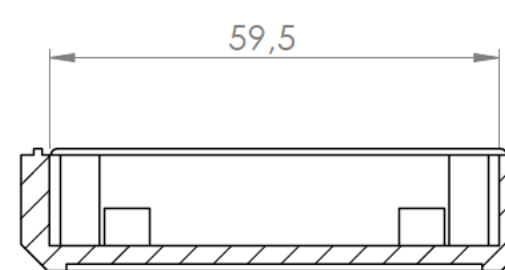
Sección/ Section W-W
