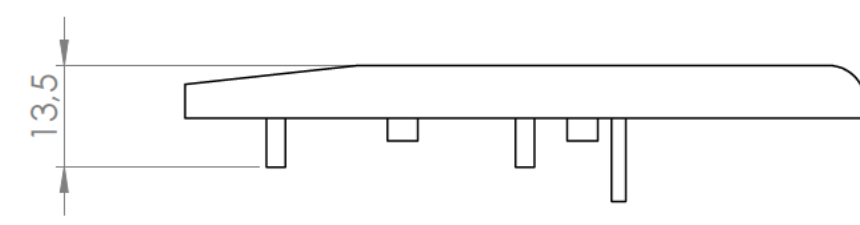
Sección M-M / Section M-M
