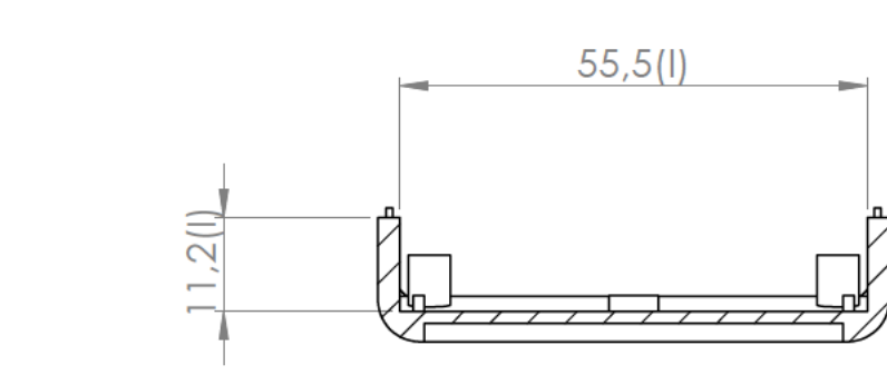
Sección Q-Q/Section Q-Q
