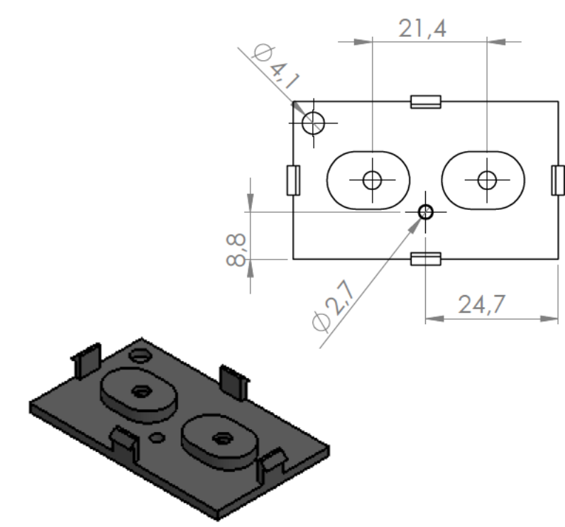
Tapeta botones Botoom door
