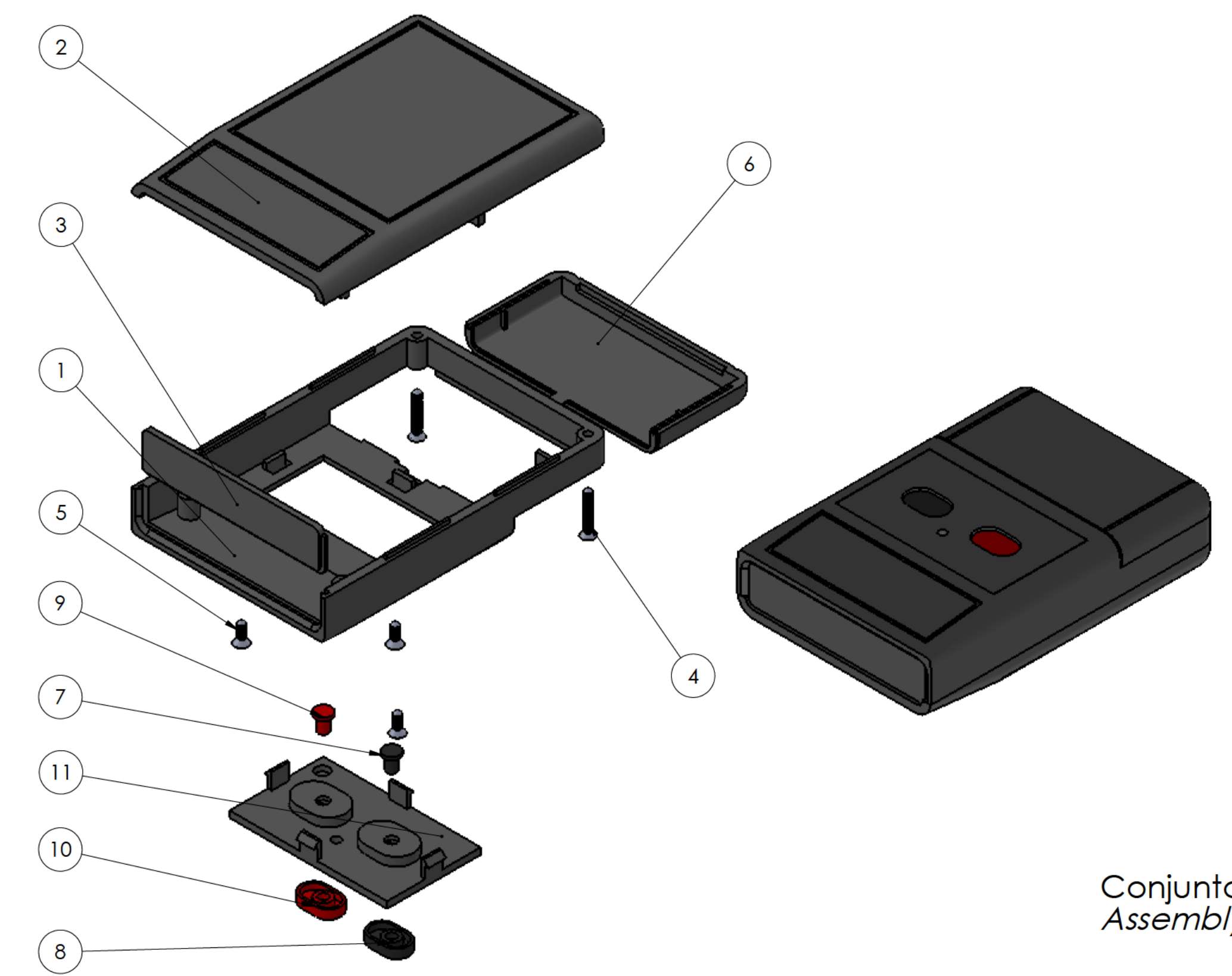
Tapeta botones Botoom door
