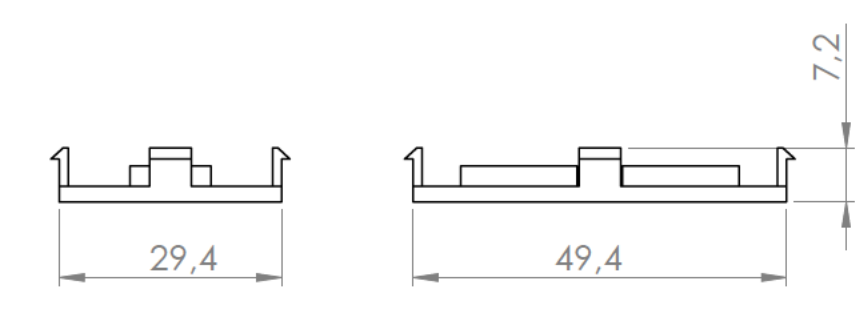
Tapeta posterior Botoom door
