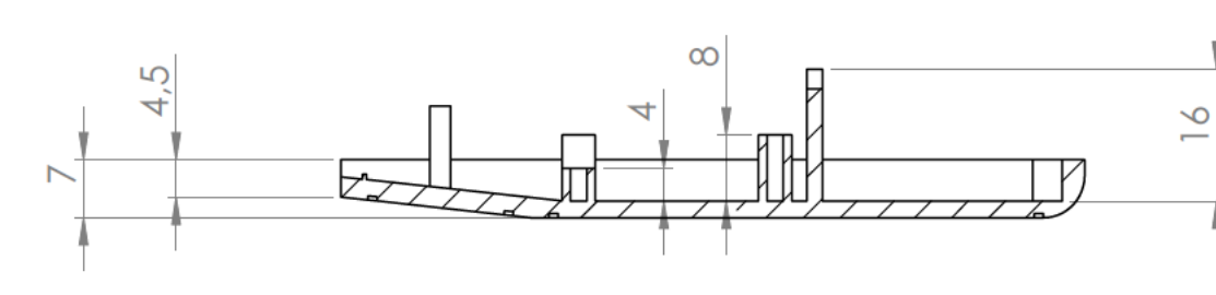
Sección M-M / Section M-M
