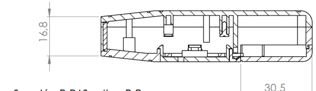
Sección P-P/Section P-P
