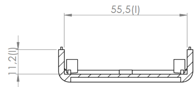
Sección Q-Q/Section Q-Q
