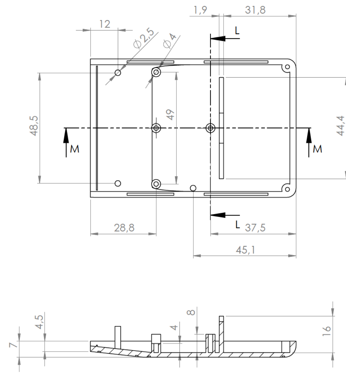
Sección M-M / Section M-M
