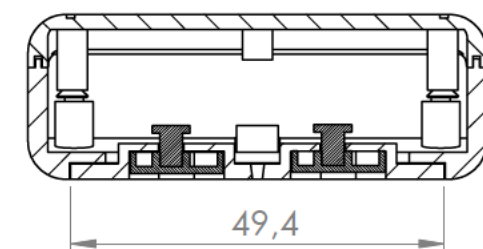
Sección/Section R-R
