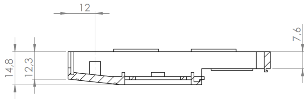
Sección N-N/Section N-N
