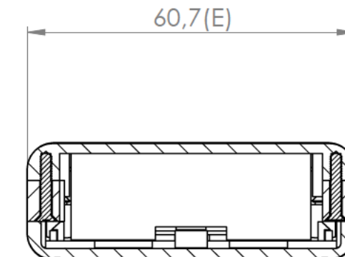
Sección S-S/Section S-S
