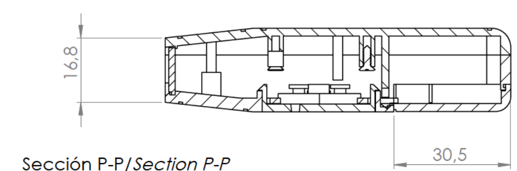
Sección P-P/Section P-P
