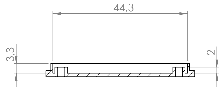
Sección/Section AC-AC
