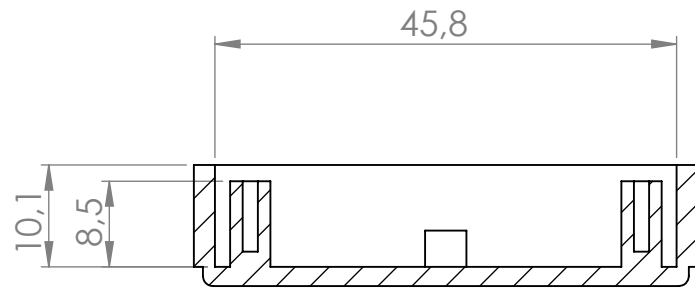
Sección/Section AF-AF
