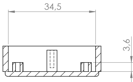
Sección/Section AG-AG
