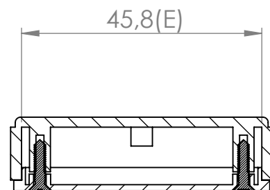
Sección/Section A-A
