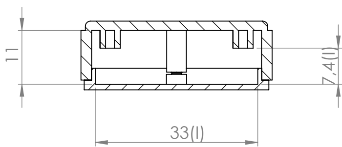
Sección/Section AH-AH
