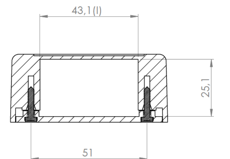
Sección /Section M-M
