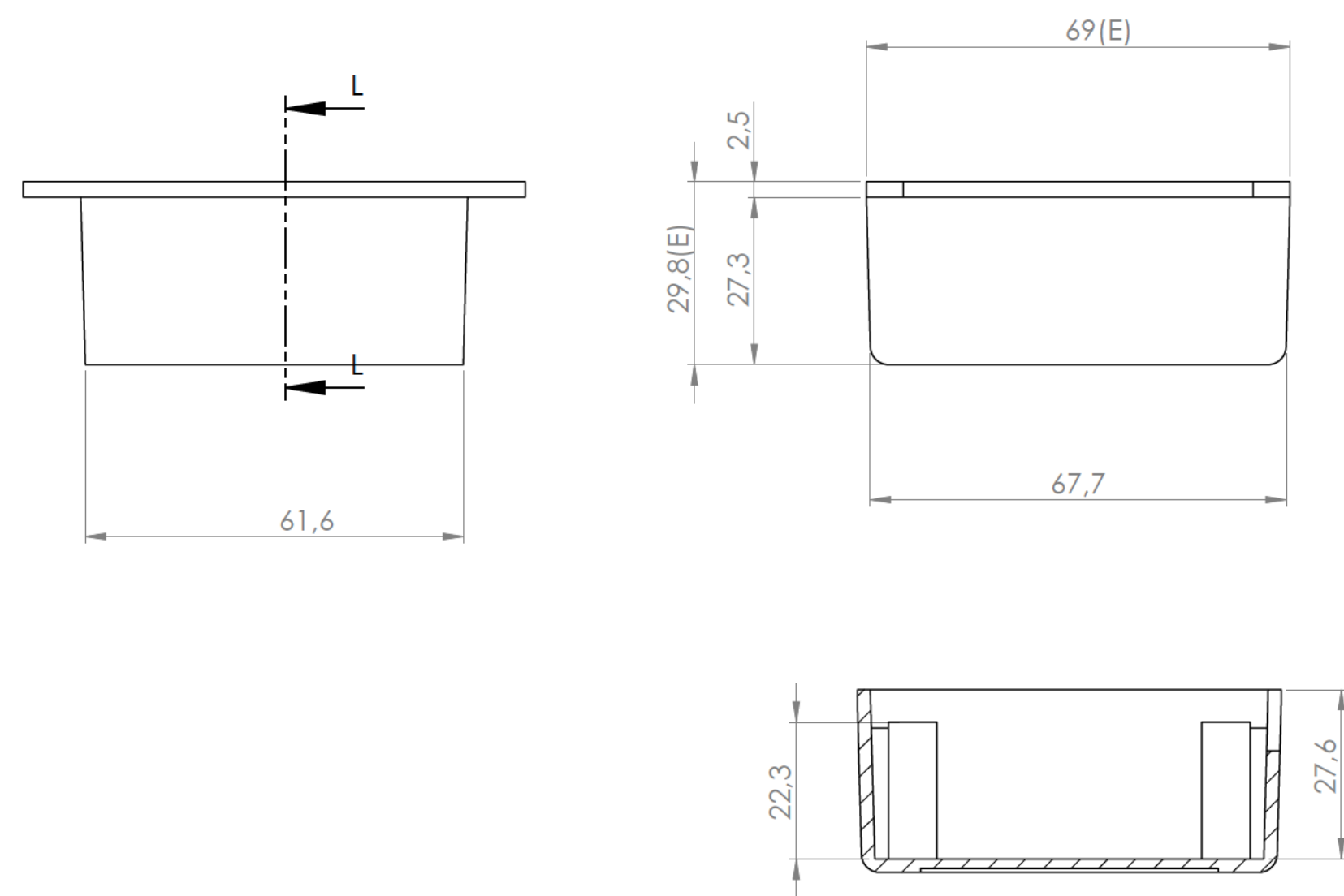
Sección /Section L-L
