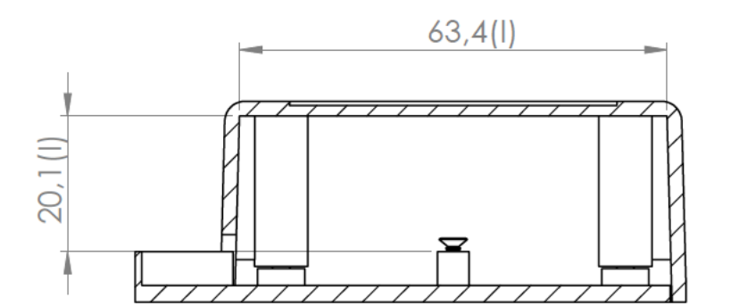
Sección /Section P-P
