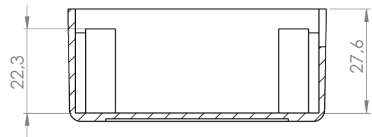
Sección /Section L-L
