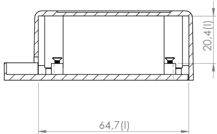
Sección /Section M-M
