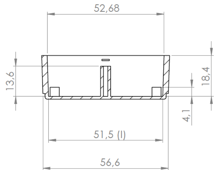
Sección/Section D-D
