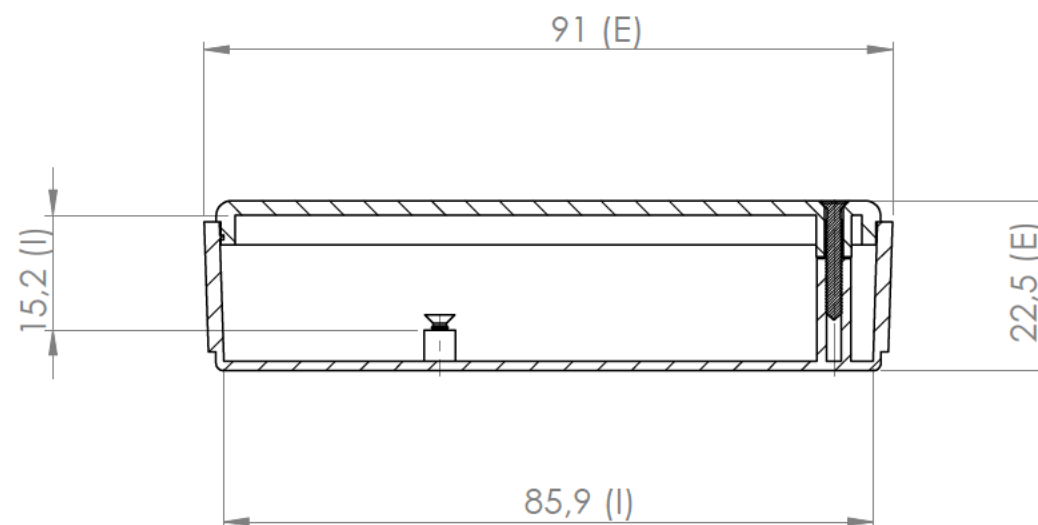
Sección/Section G-G
