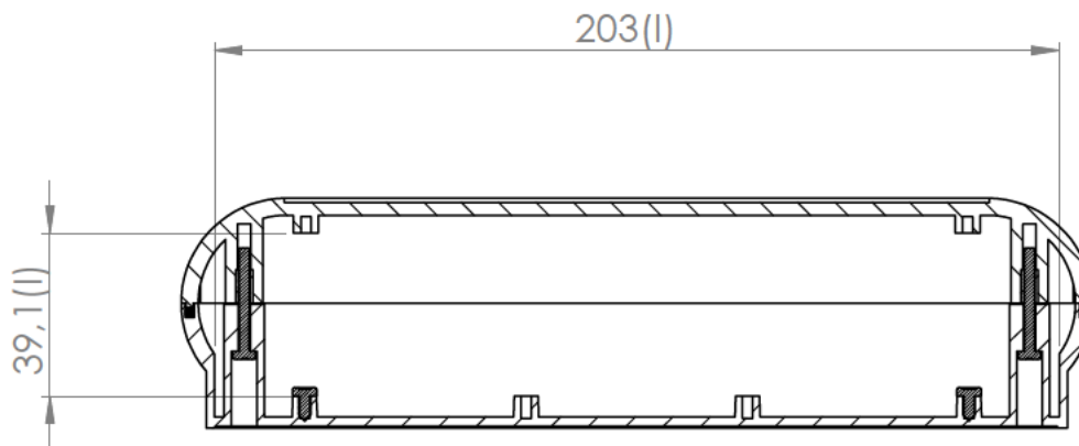
Sección / Section O-O
