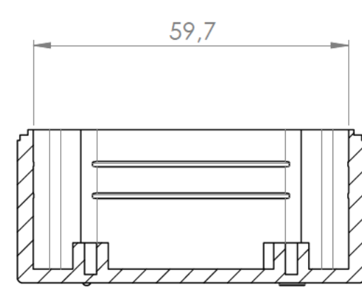
Sección/Section T-T Escala/Scale
