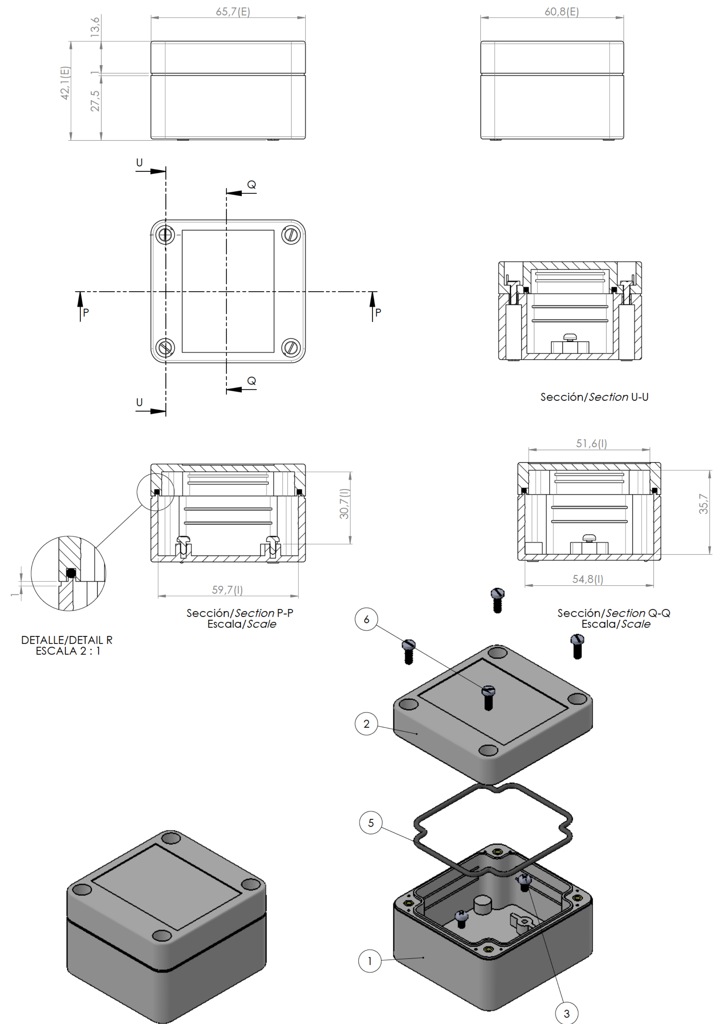
Conjunto Assembly
