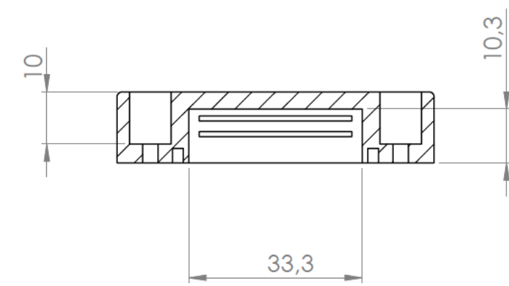
Sección/Section L-L Escala/Scale
