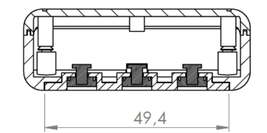
Sección R-R / Section R-R
