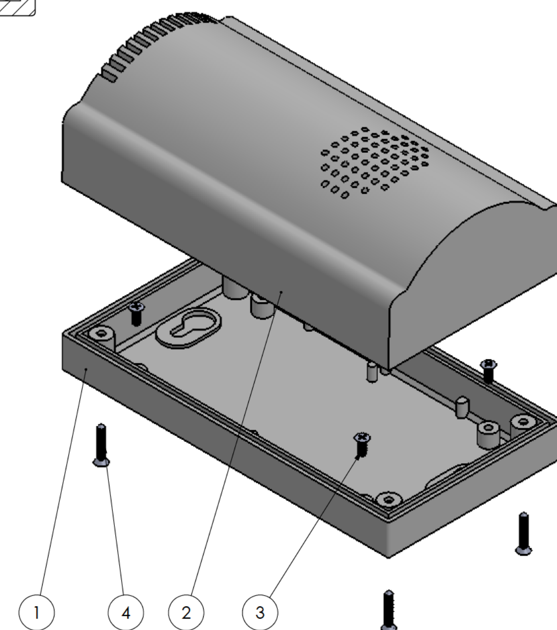
Conjunto Assembly
