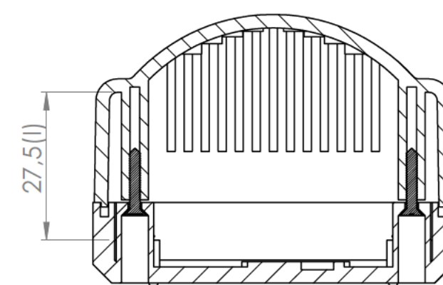
Sección/Section P-P
