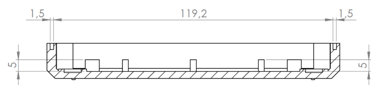
Sección/Section M-M
