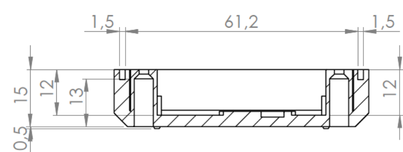
Sección/Section L-L
