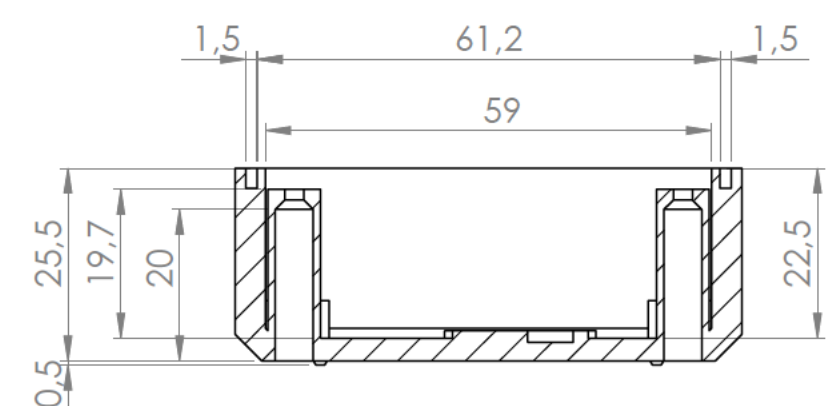
Sección/Section L-L
