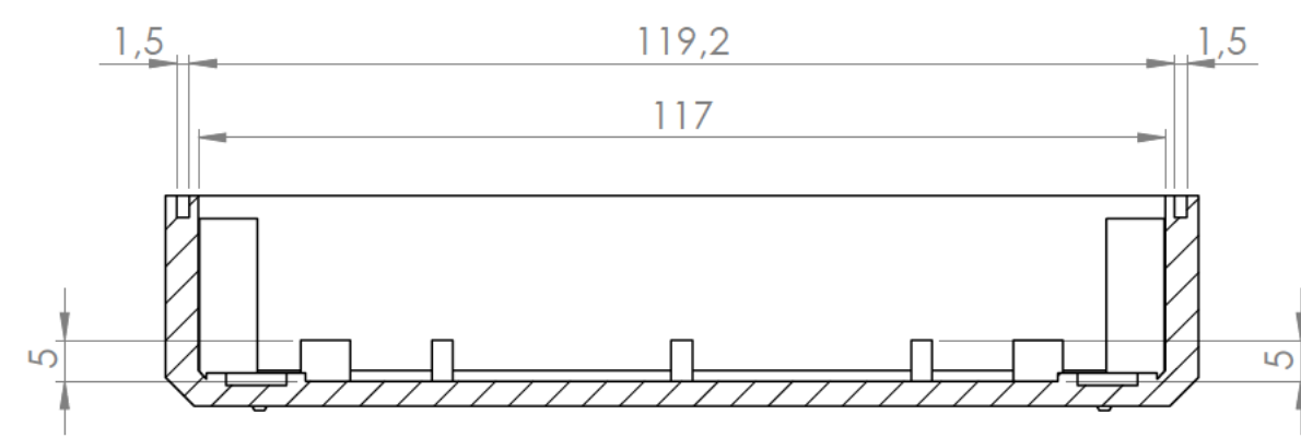
Sección/Section M-M
