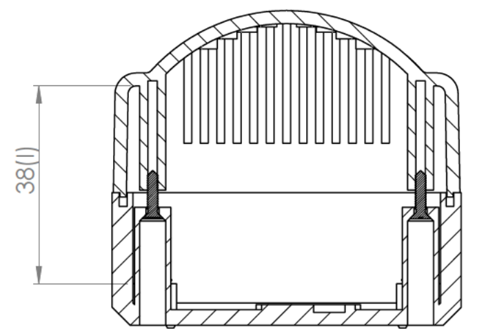
Sección/Section P-P
