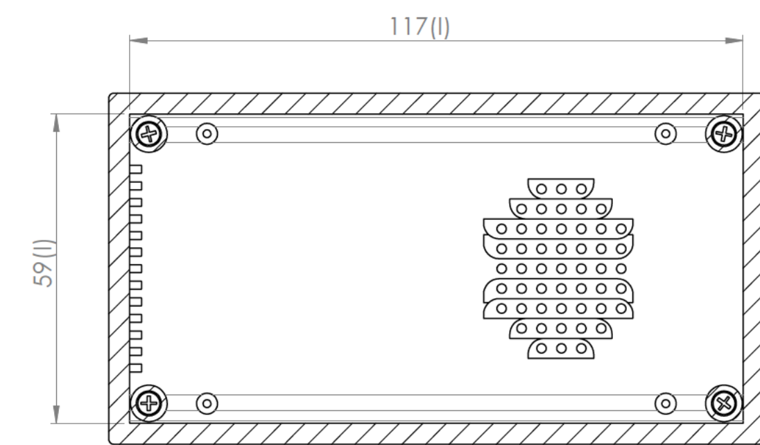
Sección/Section Q-Q
