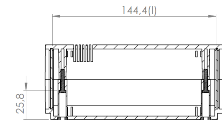
Sección/Section M-M
