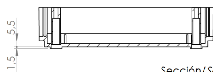
Sección/Section L-L
