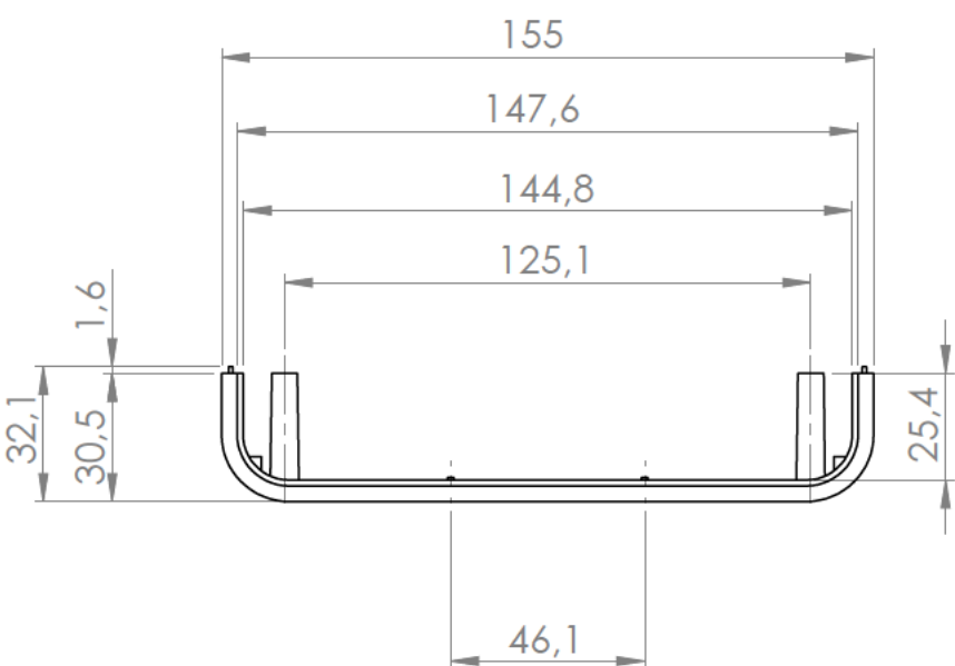
Sección/Section L-L
