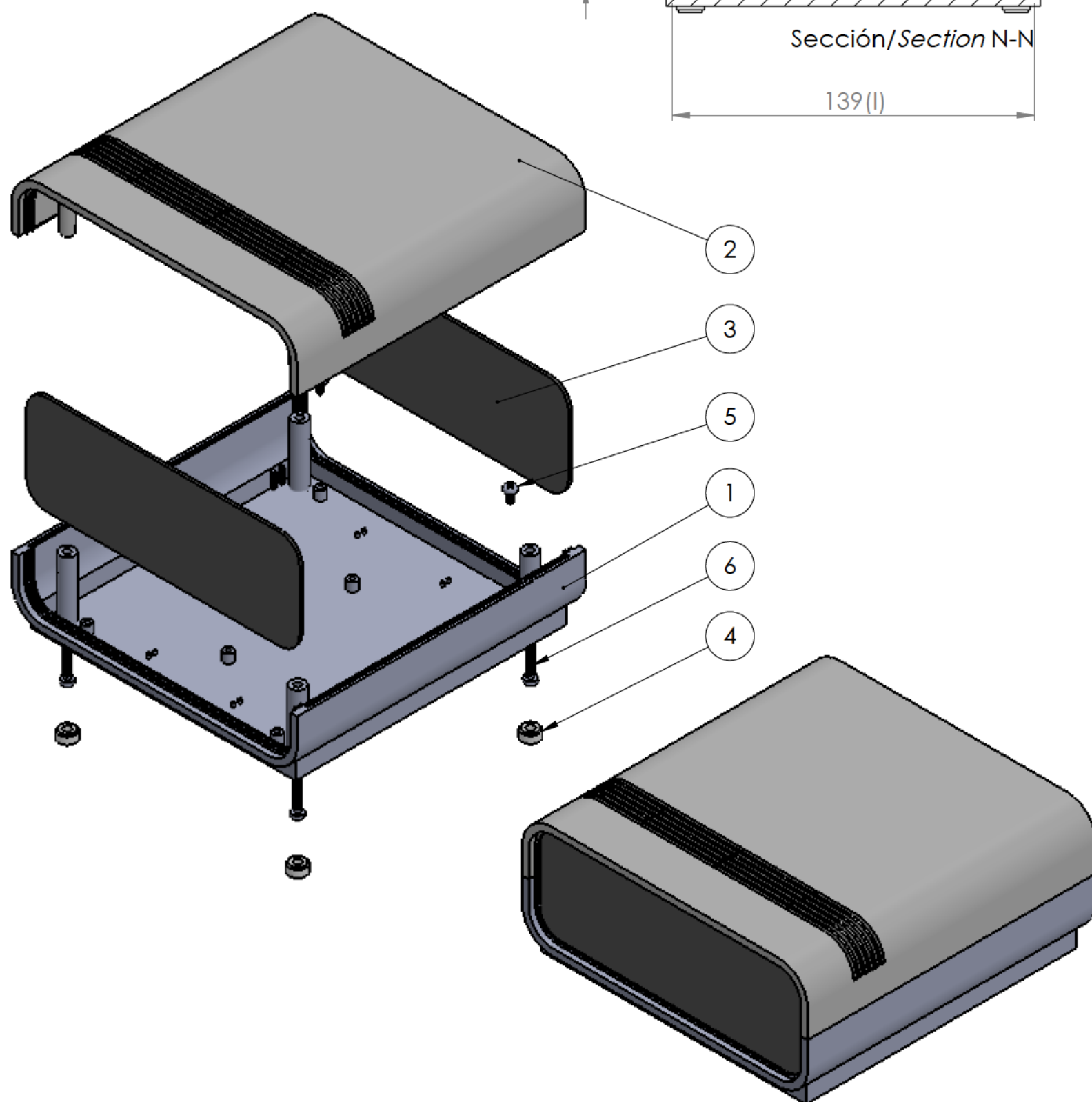
Conjunto Assembly
