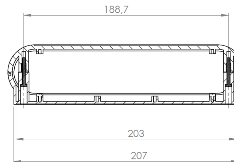
Sección/Section M-M
