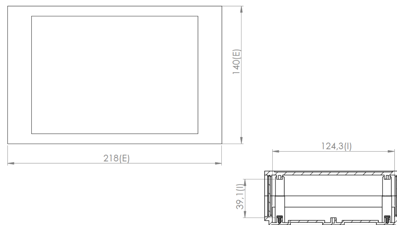
Sección/Section L-L
