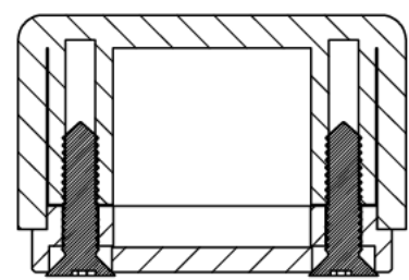
Sección/ Section U-U
