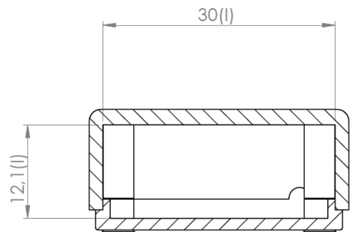
Sección/ Section V-V
