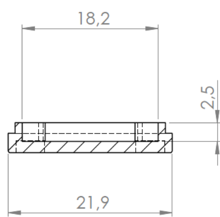
Sección/ Section Y-Y
