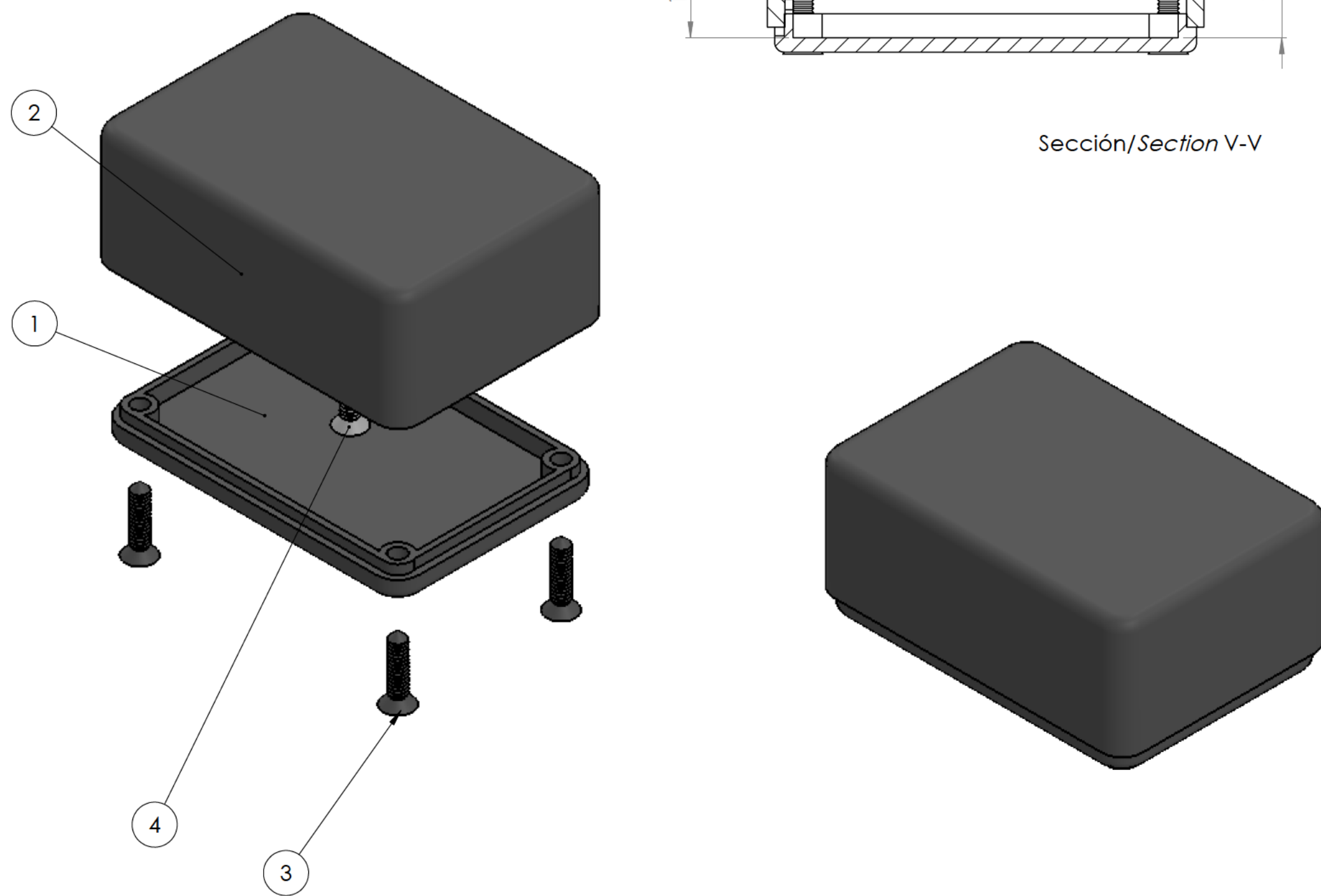
Conjunto Assembly
