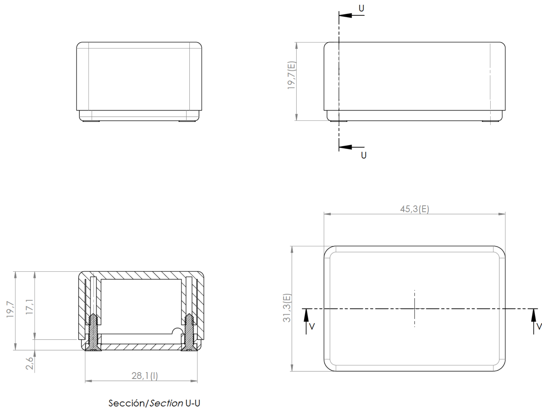
Sección/Section U-U
