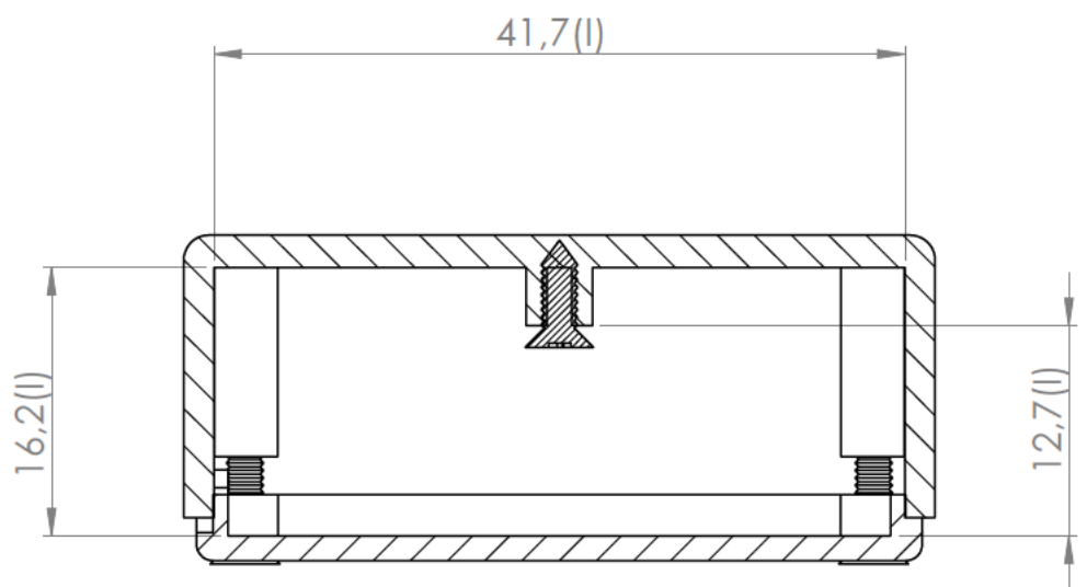
Sección/Section V-V
