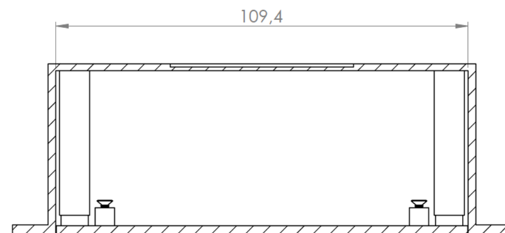
Sección/Section O-O
