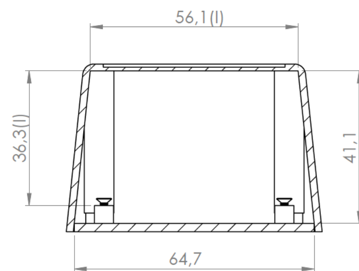
Sección/Section N-N
