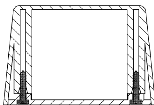
Sección/Section L-L
