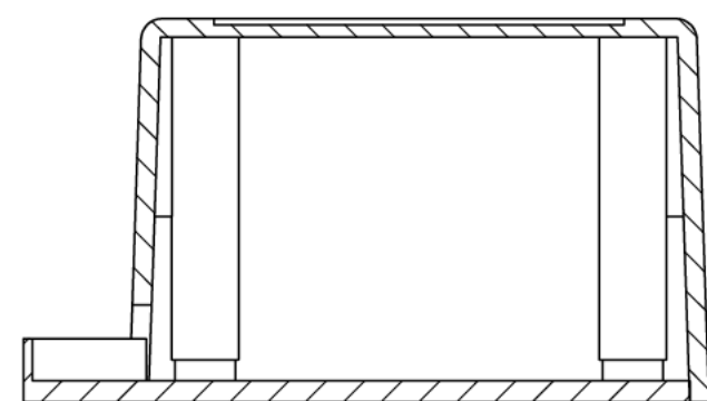
Sección /section P-P
