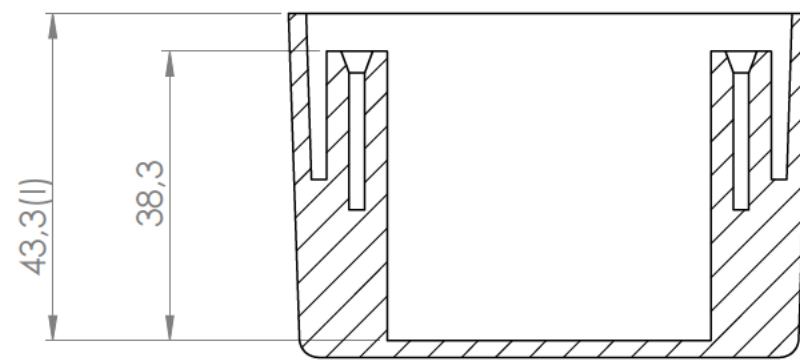
Sección / Section L-L
