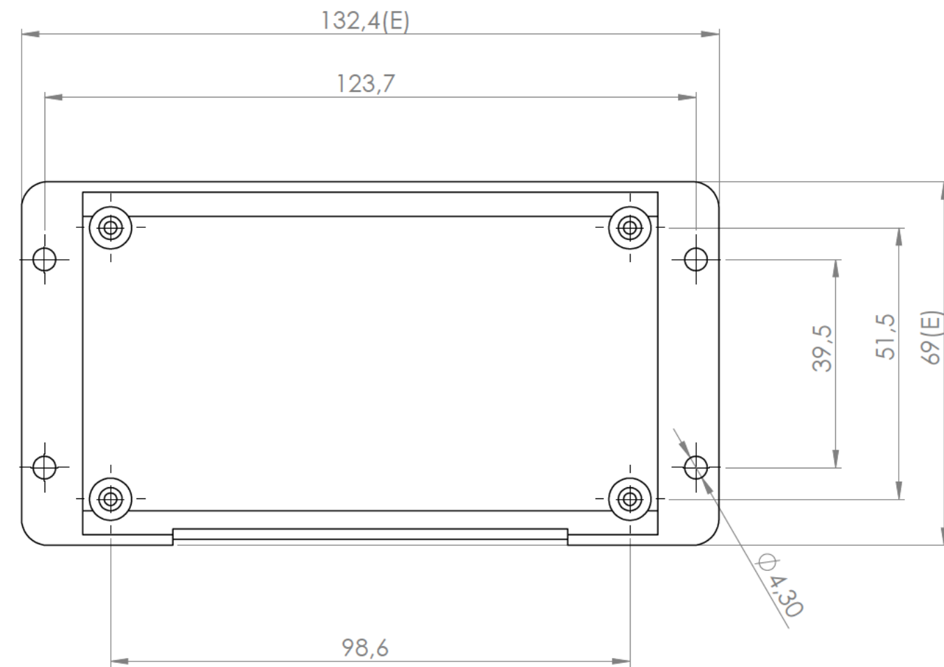
Sección/ Section M-M
