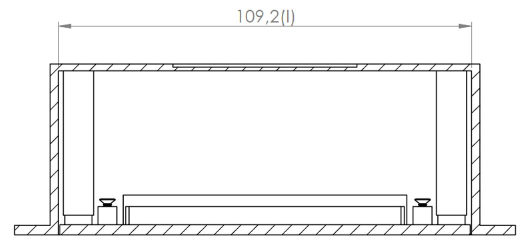
Sección/ Section O-O
