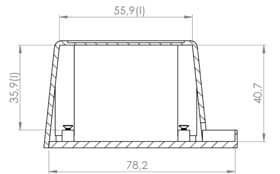
Sección/ Section N-N
