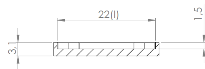
Sección/Section K-K
