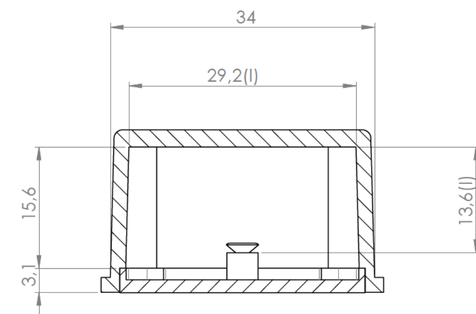
Sección/Section O-O
