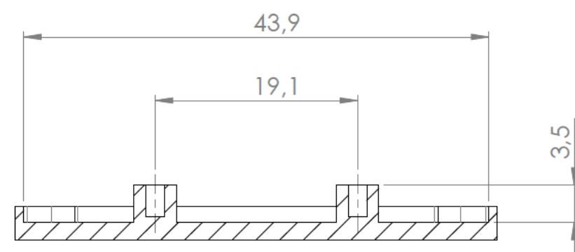
Sección/ Section P-P
