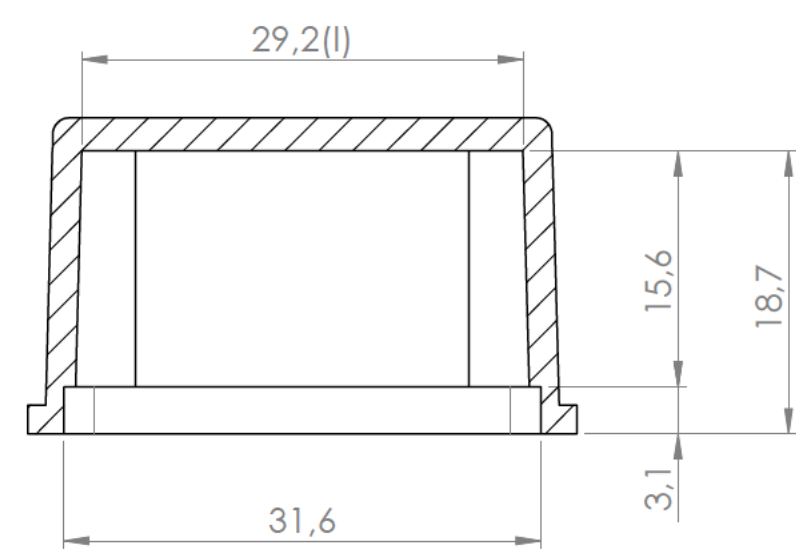
Sección/Section L-L
