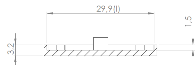
Sección/Section K-K
