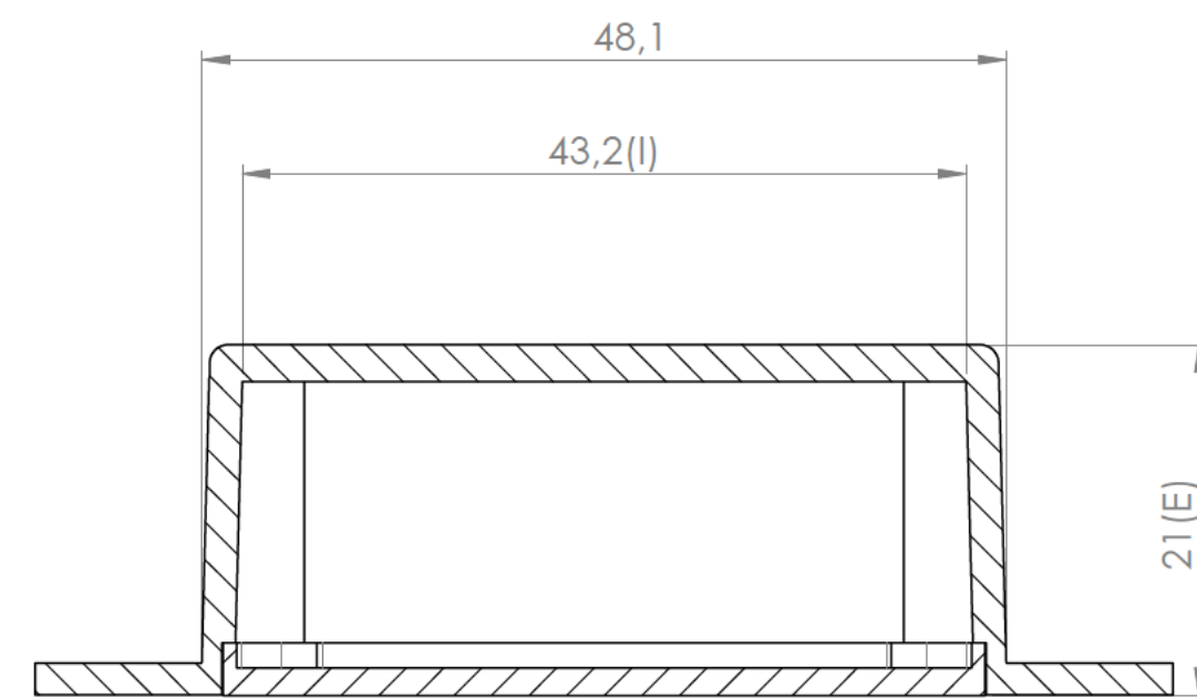
Sección/Section N-N
