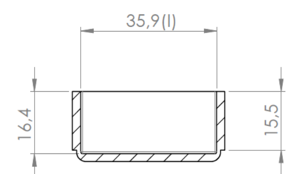
Sección/Section S-S
