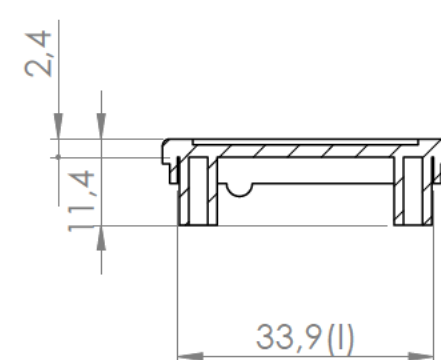
Sección/Section L-L
