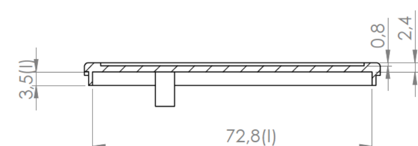
Sección/Section M-M
