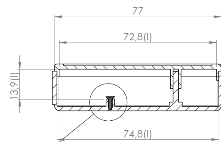
Sección/Section P-P
