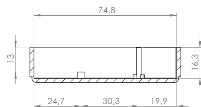
Sección/Section T-T
