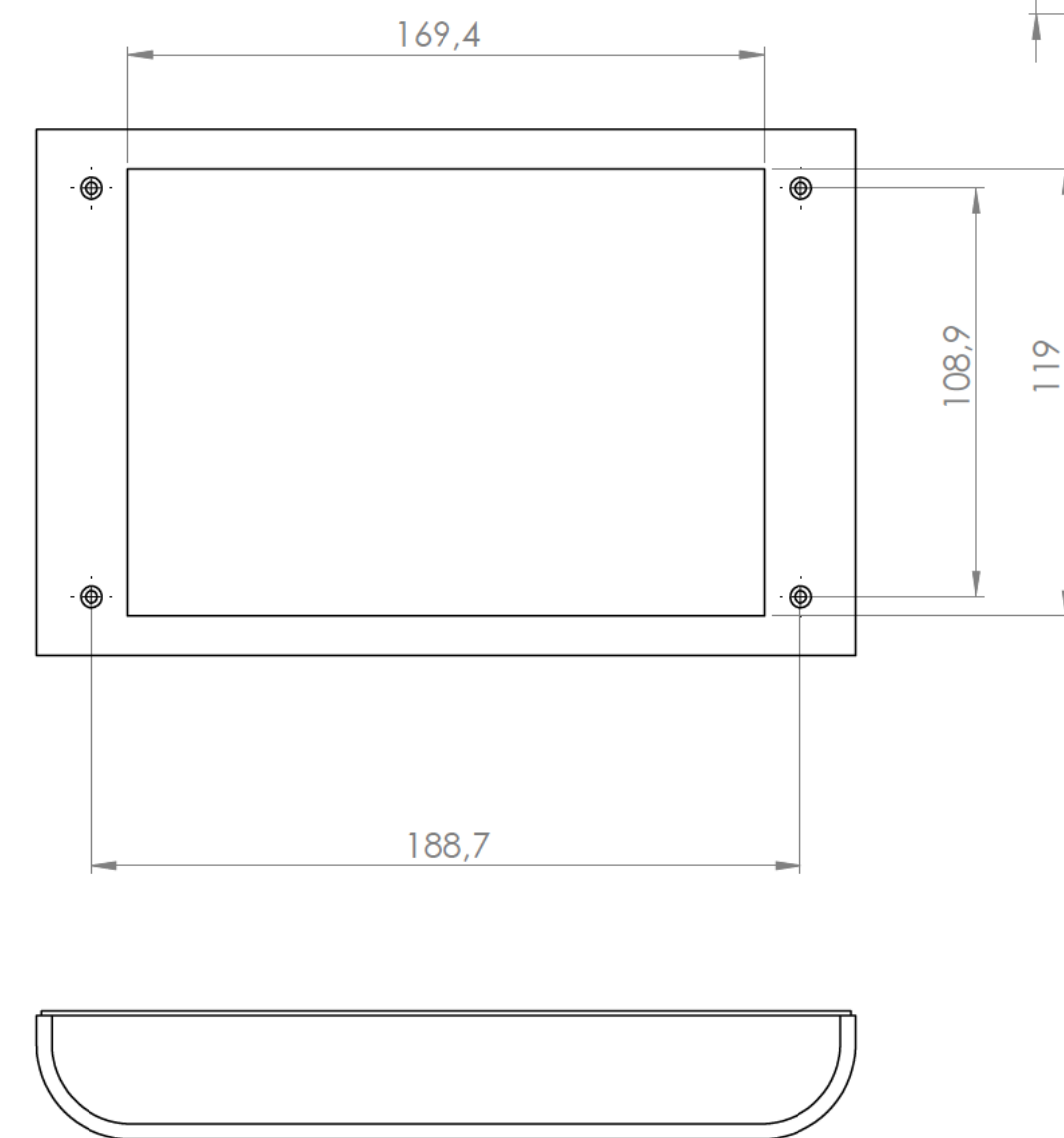
Sección/ Sección M-M
