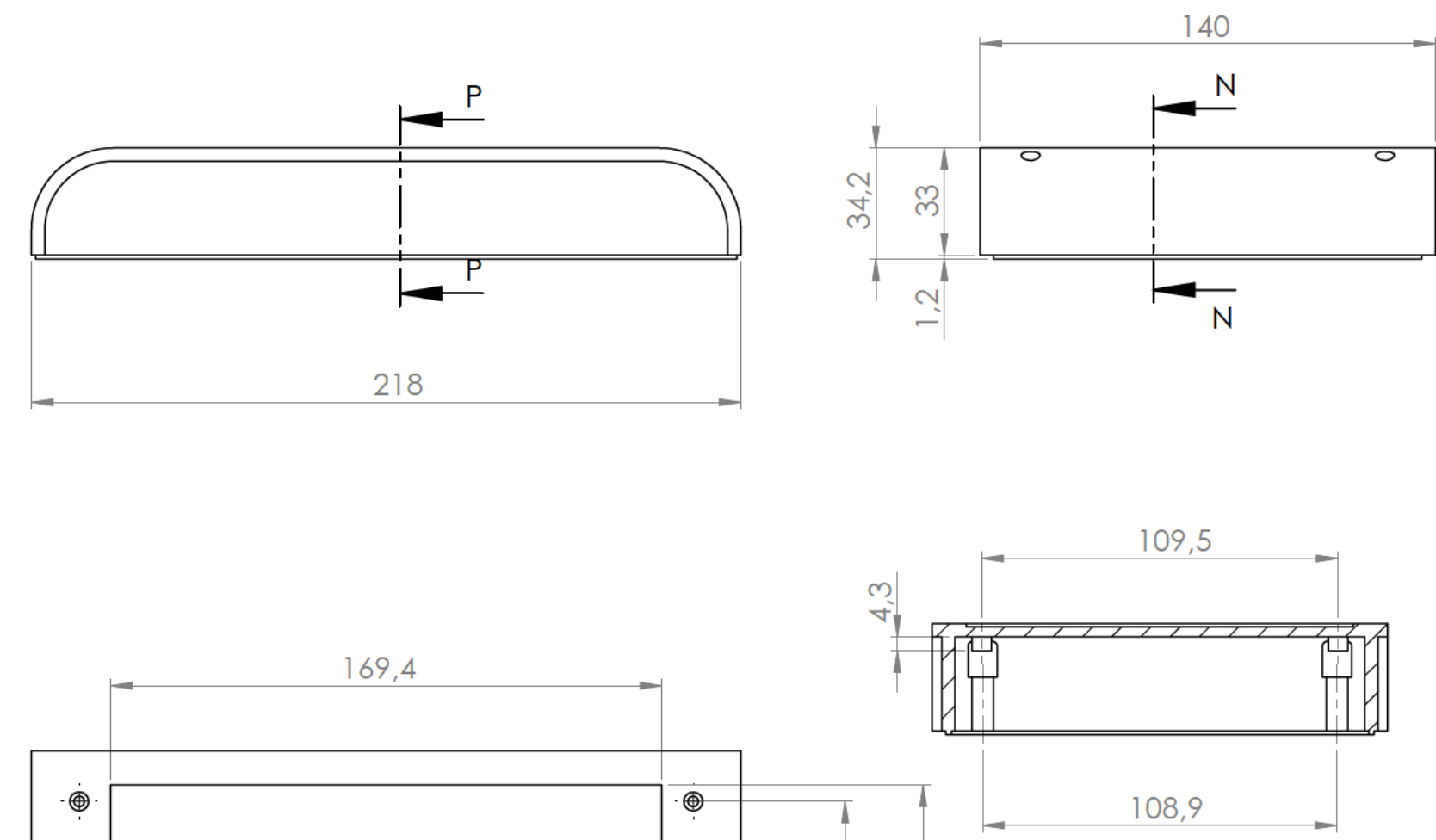
Sección / Section P-P
