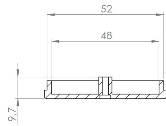
Sección/ Section W-W
