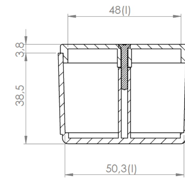
Sección/Section U-U
