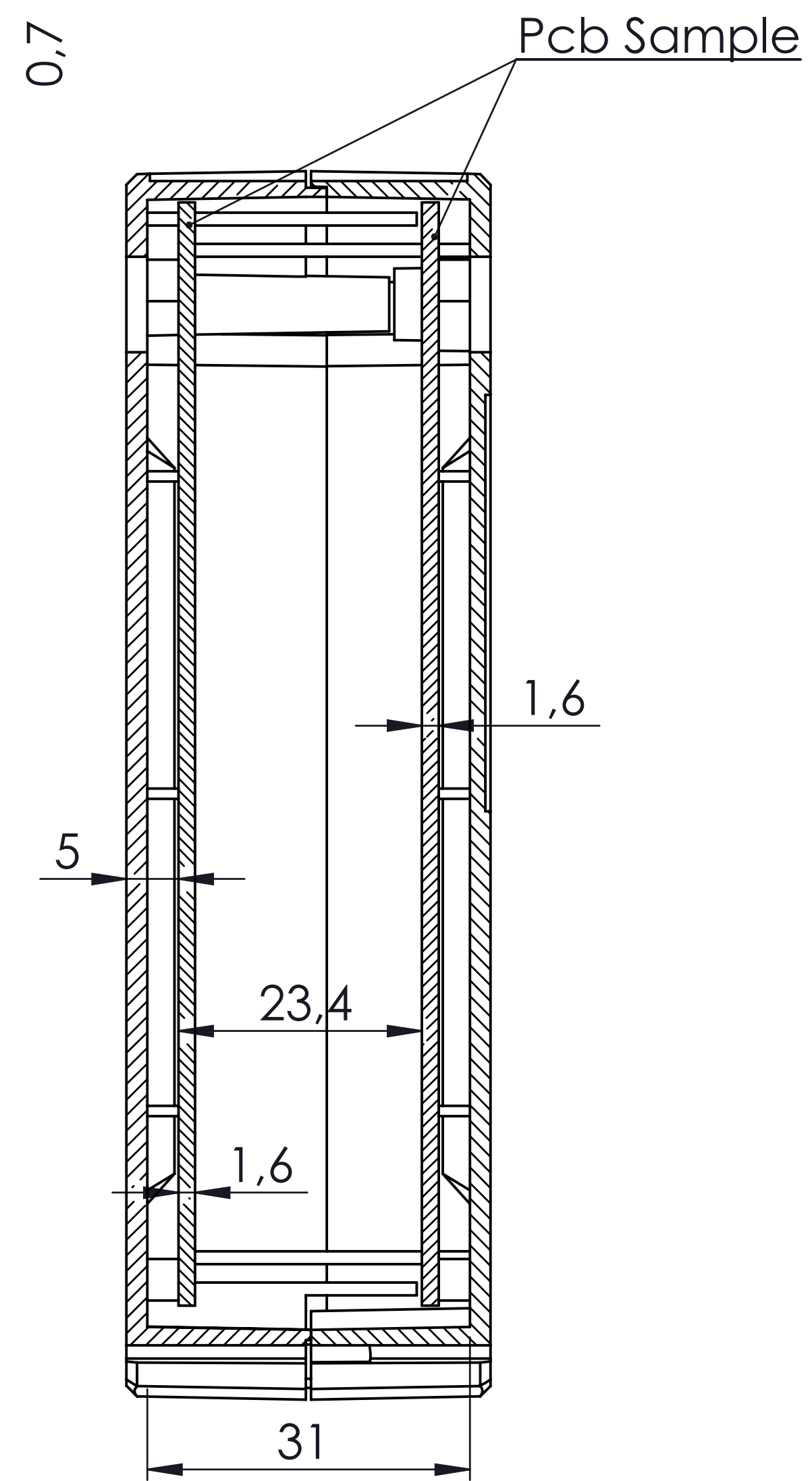
SECTION A-A
