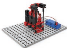
Exzenterpresse / Eccentric press / Presse à excentrique / Excentrische pers / Prensa excéntrica / Prensa excéntrica / Pressa eccentrica / Эксцентрический пресс / 偏心压力机.....126
