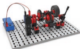
Schaltgetriebe - 2 Gang / Manual gearbox - 2 gear / Boîte de vitesses manuelle - 2 rapports / Handgeschakelde versnellingsbak - 2 versnellingen / Caja de cambios manual - 2 marchas / Caixa de velocidades manual - 2 velocidades / Cambio manuale - 2 marce / Механическая коробка передач - 2 передача / 手动变速箱--2档.....49
