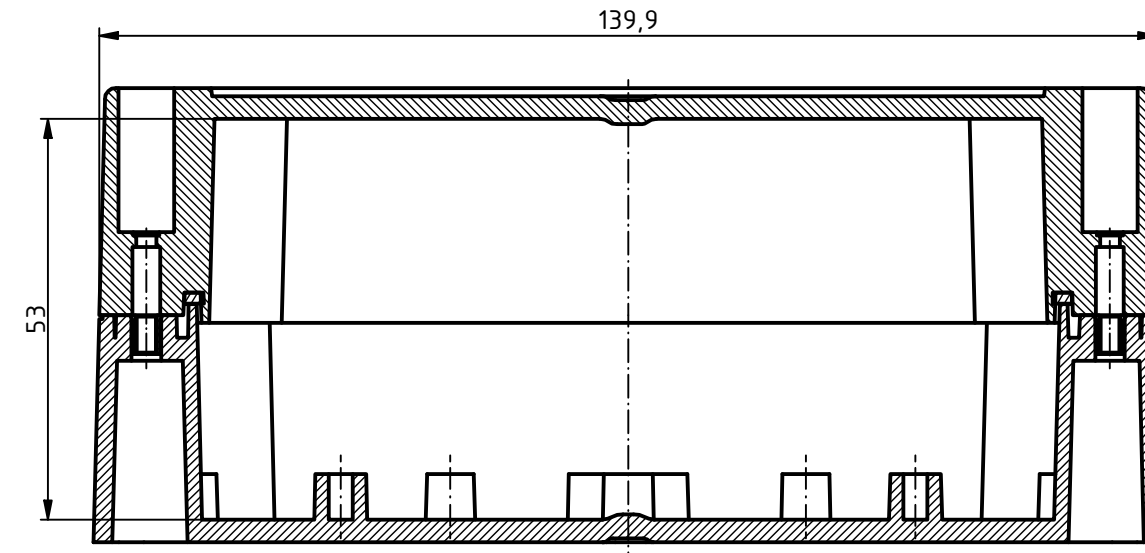
A-A ( 1 : 1 )
