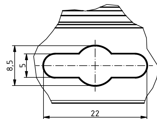
X ( 2 : 1 )
