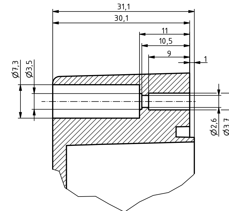
Y ( 2 : 1 )
