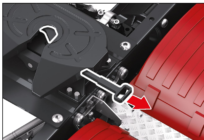
Sattelkupplung geöffnet Lock buckle open state
