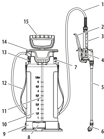
Teile des Drucksprühveräts
