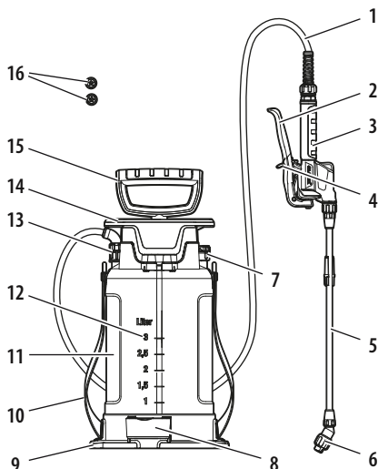
Teile des Drucksprühveräts
