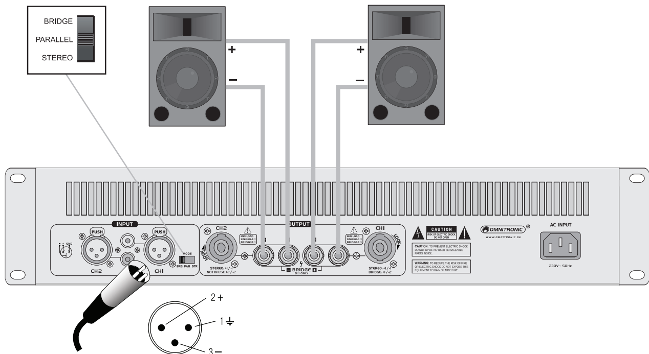
Abb. 6 Verwendung der Schraubklemmen im Brückenbetrieb
