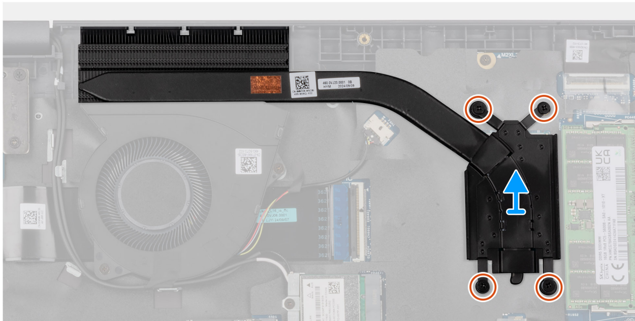
Abbildung 43. Kühlkörper entfernen
