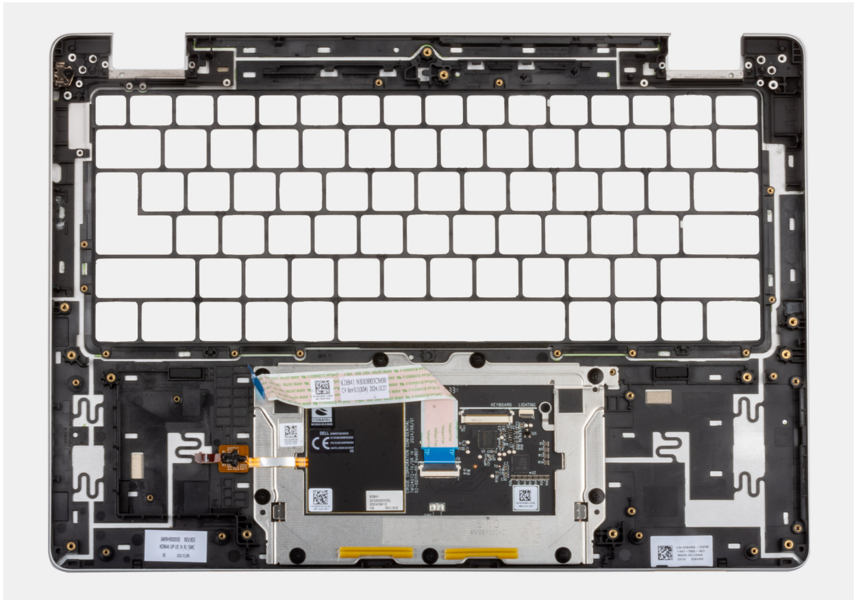
Abbildung 102. Handauflagenbaugruppe
