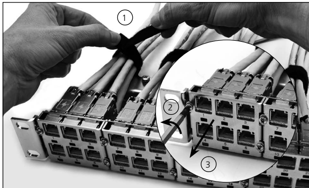
Demontage der Modulaufnahme / Demounting of module carrier
