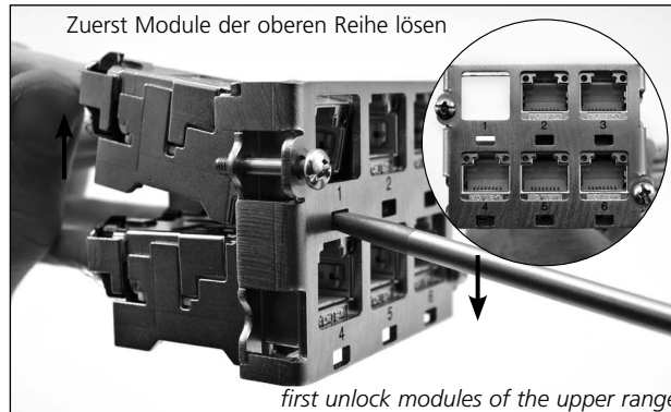
Demontage des Moduls / Demounting of module
