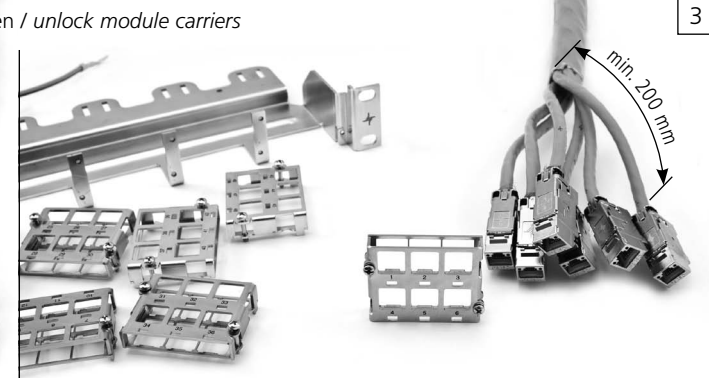
3 Modul an Kabel gemäß Montagehinweis B05030A0267 anschließen / connect module to cable according to mounting information B05030A0267
