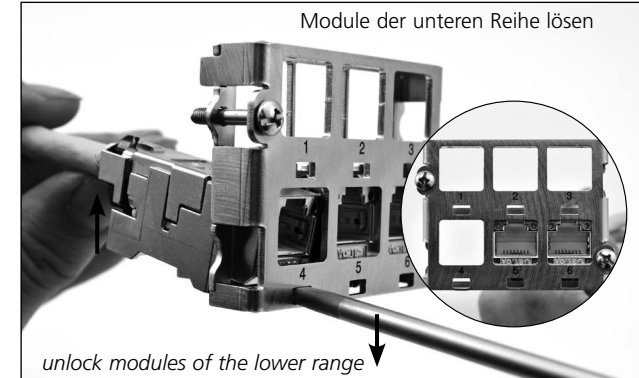
Demontage des Moduls / Demounting of module
