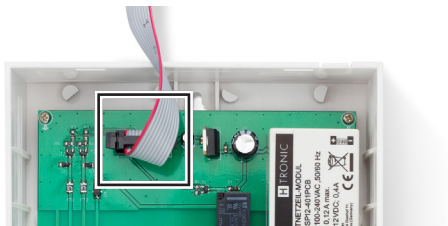
Abbildung 16 Displaykabel entfernen
