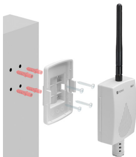
Abbildung 8 Halterung Funk-Luftfeuchtesensor; Montage an Wand
