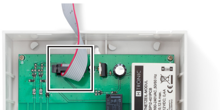
Abbildung 17 Displaykabel befestigen
