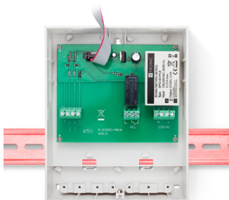
Abbildung 7 Montage Hutschienen
