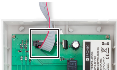
Abbildung 22 Displaykabel befestigen
