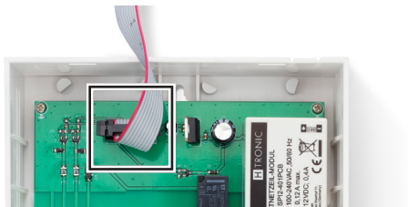
Abbildung 20 Displaykabel entfernen
