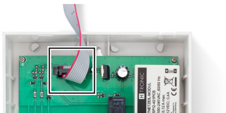
Abbildung 6 Displaykabel befestigen
