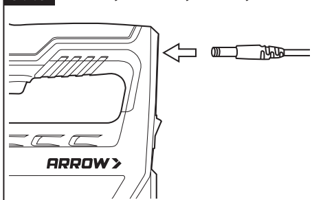
Obr. 9 Vložte nabíjačku do zadnej časti nástroja
