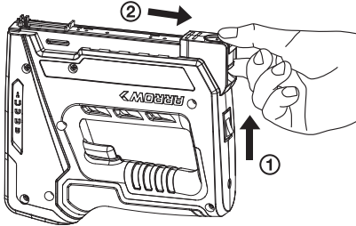
Figure.2 Chargeur à chargement par le bas à dégagement rapide
