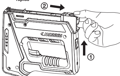
Fig. 2 Magazin de încărcare inferioară cu eliberare rapidă
