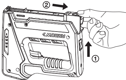
Abb. 2 Schnellverschluss-Bodenladermagazin
