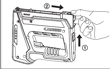
Fig.2 Revista De Carga Inferior De Liberación Rápida
