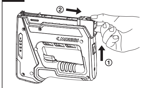
Obr. 2 Rýchlopínací zásobník so spodným plnením
