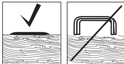
Fig. 8 a: agrafă fixată corespunzător b: agrafă fixată necorespunzător
