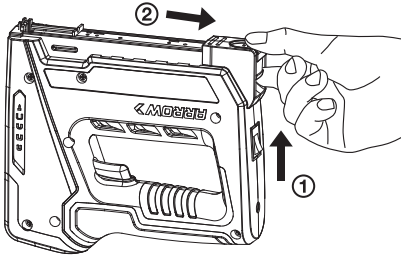
Rys. 2 Szybkozłączka magazynka ładowanego od dołu
