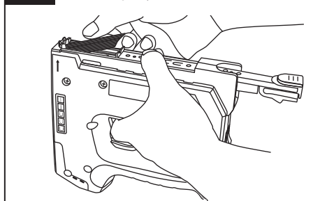
Obr. 4 Umiestnite sponky do kanála, nožičkami hore
