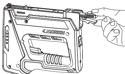
Sl. 3 Izvlecite potisni sklop
