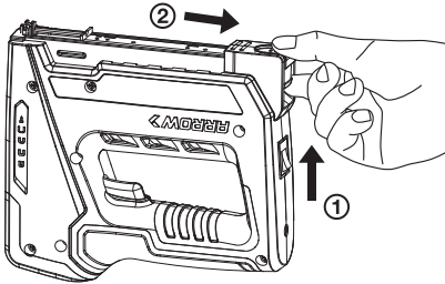
Fig. 2 Hurtigudløsende bundmagasin
