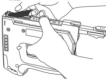
Fig. 4 Așezați capsule în canal, cu partea inferioară în sus
